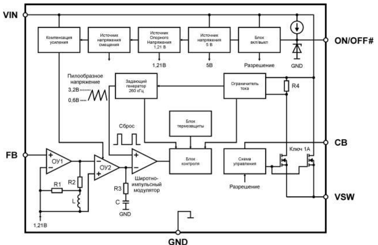
Рисунок 15 – Структурная схема микросхемы 1273PIN1T1
