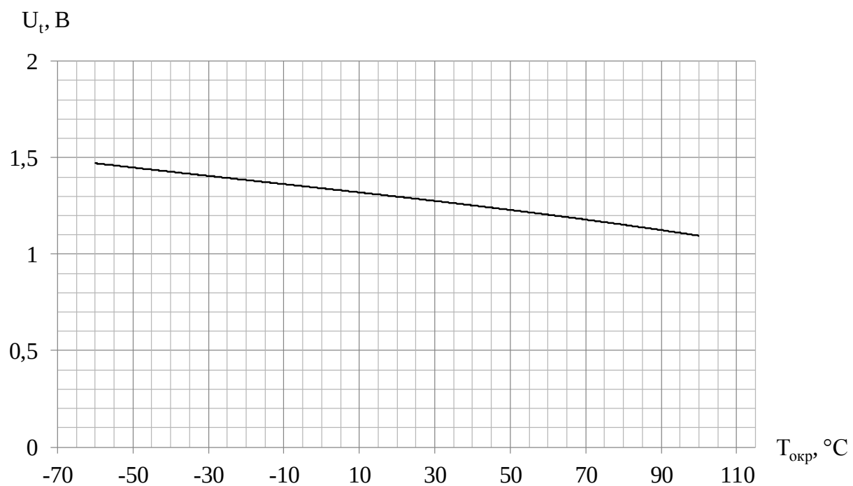
Рисунок 10 – Зависимость порогового напряжения по входу ON/OFF# от температуры окружающей среды при U_{\text{IN}} = 12 \text{ В} , I_{\text{LOAD}} = 0,1 \text{ А}
