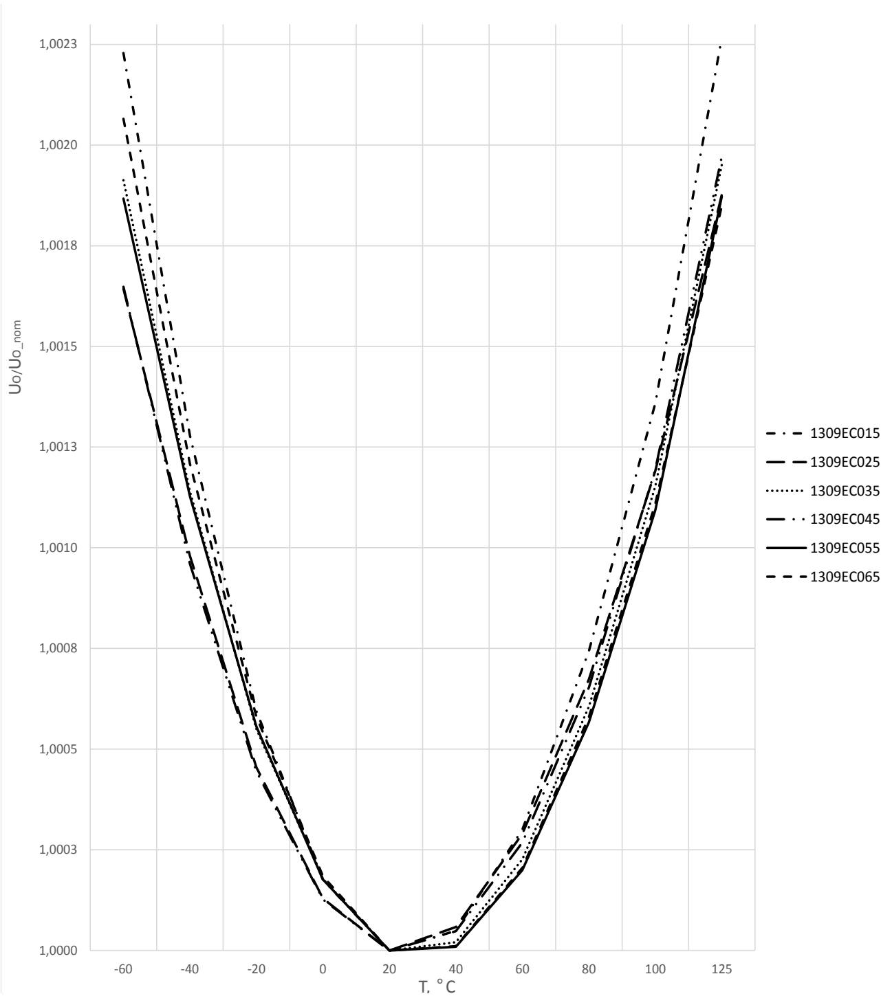
Рисунок 13 – Зависимость выходного напряжения U_o , приведенного к выходному напряжению U_{o\_nom} при T = 20^\circ\text{C} , от температуры среды
