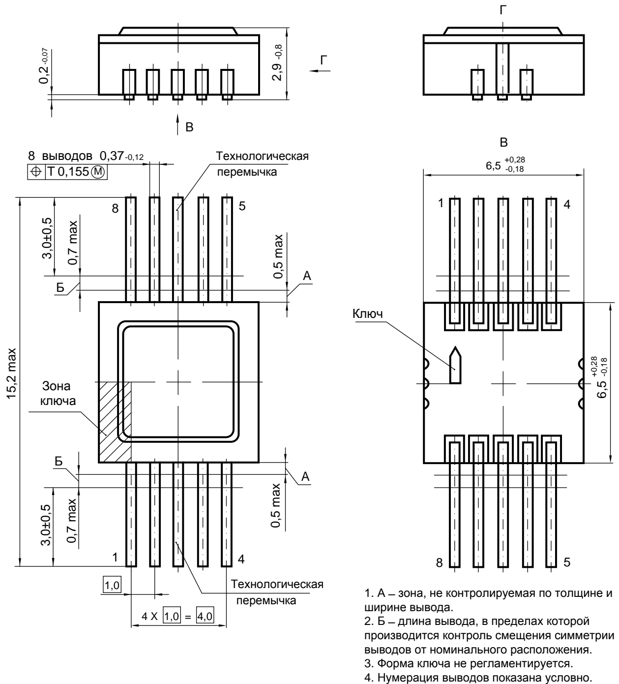
Рисунок 21 – Микросхема в корпусе H02.8-1B
