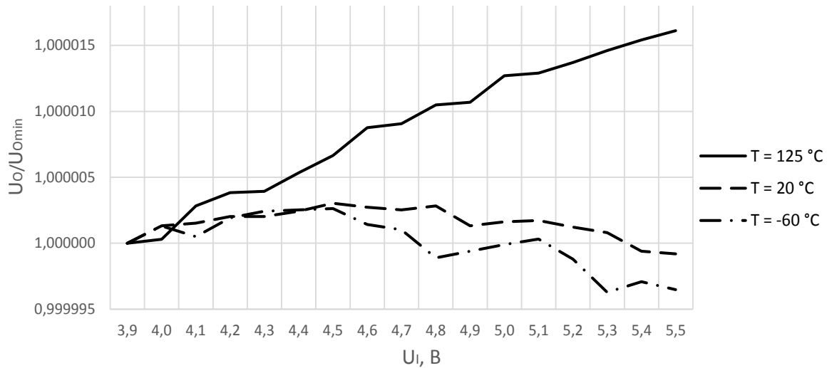
Рисунок 18 – Относительное изменение выходного напряжения U_o при изменении входного напряжения U_i при T = 20\text{ °C} микросхем 1309ЕС055
