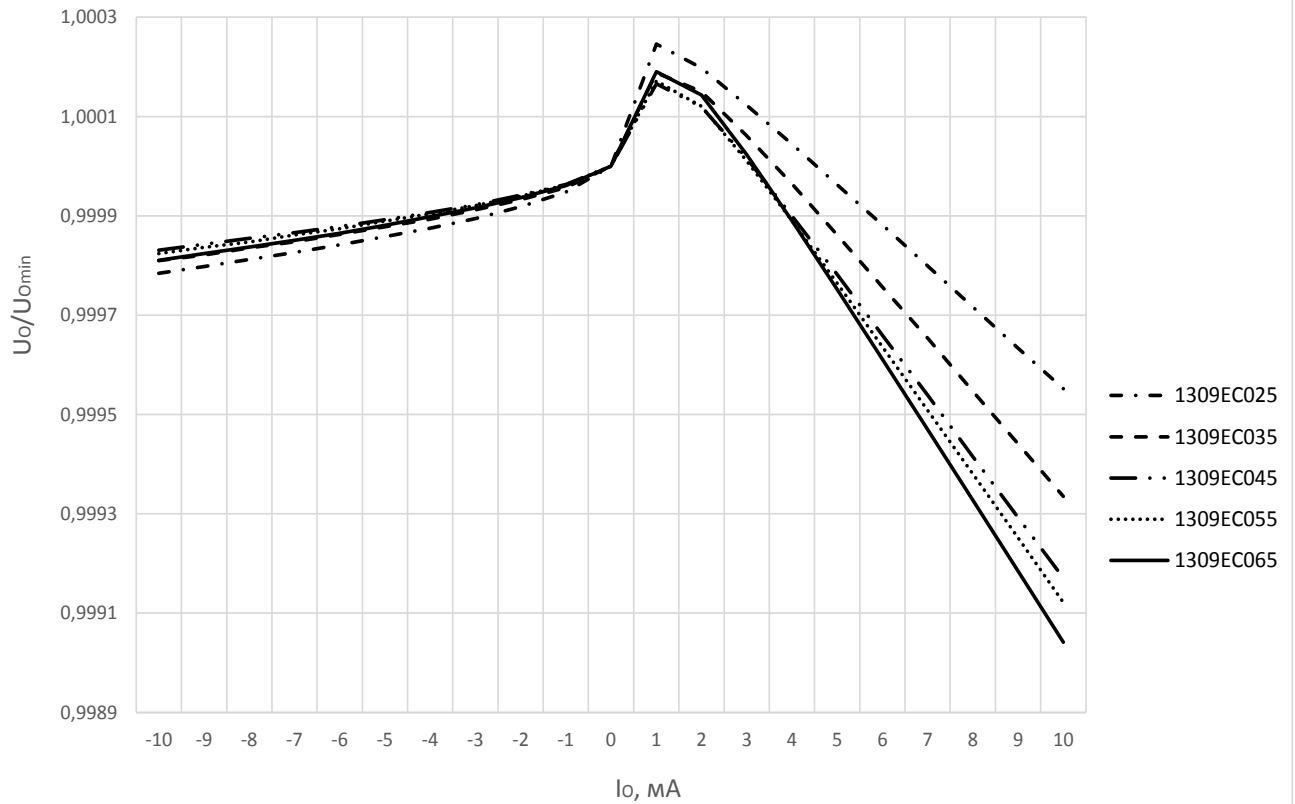
Рисунок 11 – Зависимость выходного напряжения U_o , приведенного к выходному напряжению U_{o\min} при нулевом токе нагрузки, от тока нагрузки I_o при T = 20^\circ\text{C} микросхем 1309EC025, 1309EC035, 1309EC045, 1309EC055, 1309EC065
