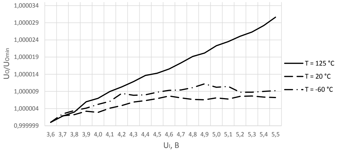
Рисунок 17 – Относительное изменение выходного напряжения U_o при изменении входного напряжения U_i при T = 20\text{ °C} микросхем 1309ЕС045
