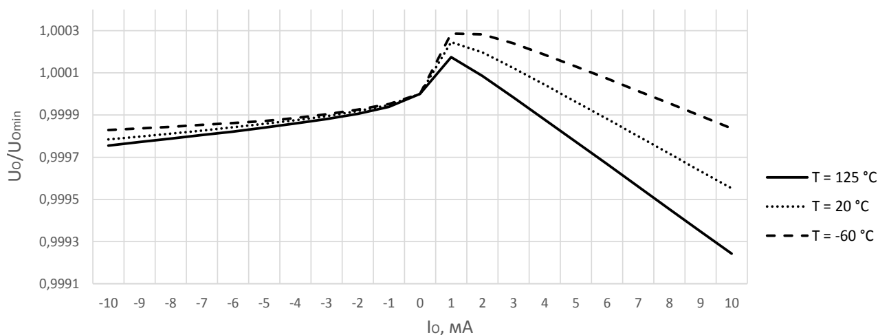
Рисунок 10 – Зависимость выходного напряжения U_o , приведенного к выходному напряжению U_{o\min} при нулевом токе нагрузки, от тока нагрузки I_o микросхем 1309ЕС025, 1309ЕС035, 1309ЕС045, 1309ЕС055, 1309ЕС065
