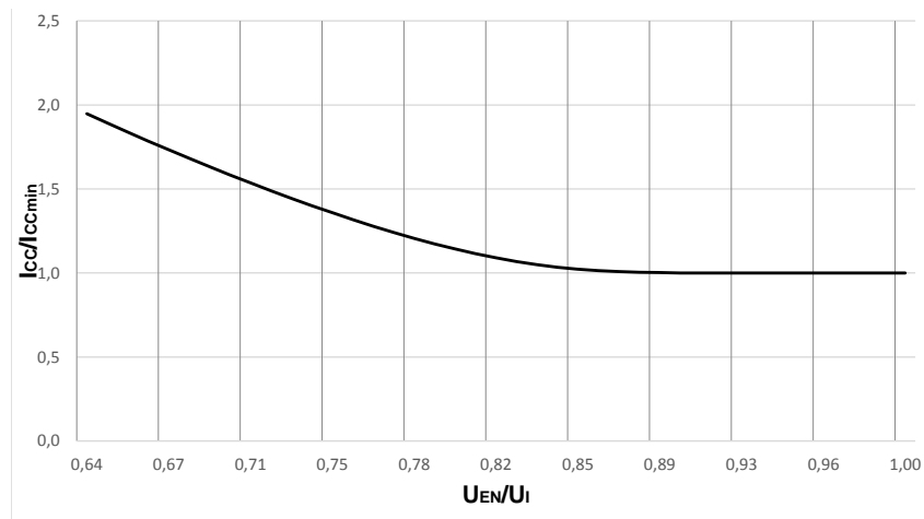
Рисунок 6 – Зависимость тока потребления I_{CC} , приведенного к току потребления I_{CCmin} при U_I = 5,5 В, от уровня сигнала EN, приведенного к U_I = 5,5 В, при T = 25^\circ\text{C}
