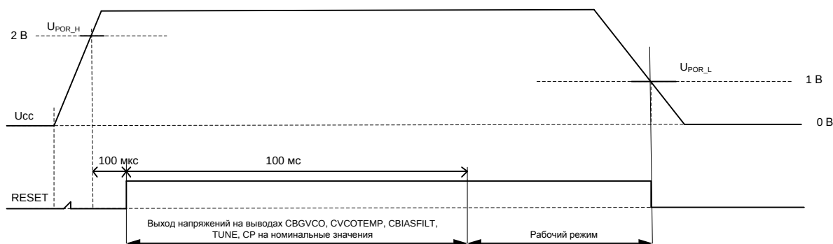
Рисунок 12 – Процедура включения и выключения микросхемы при подаче и снятии питающего напряжения
