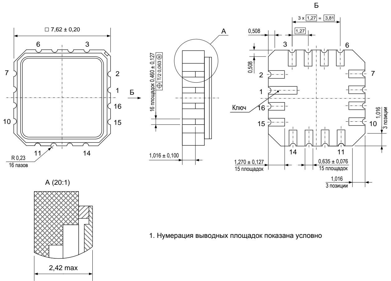
Рисунок 21 – Микросхема в корпусе 5119.16-A
