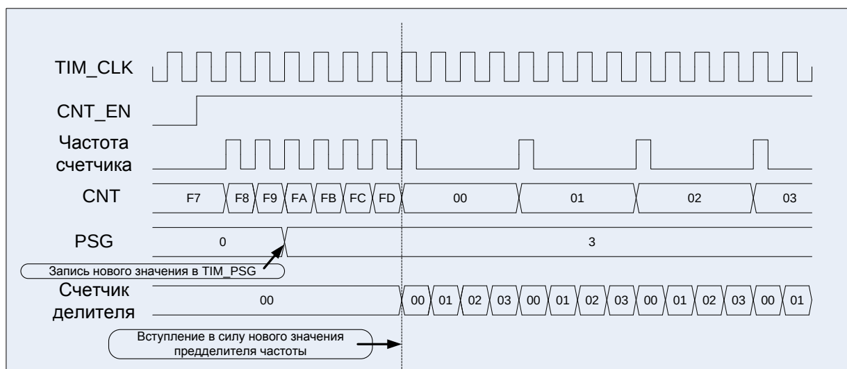
Рисунок 25 – Диаграммы работы счетчика: счет вверх
