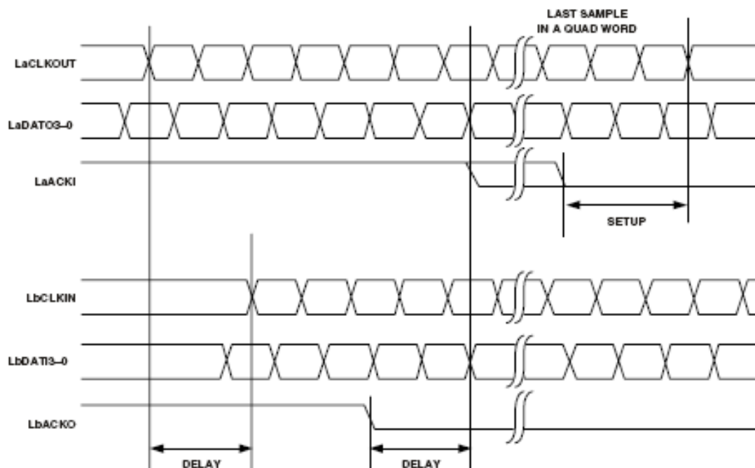
Рисунок 81 – Порт связи “а” передает порту связи “b” с задержкой
