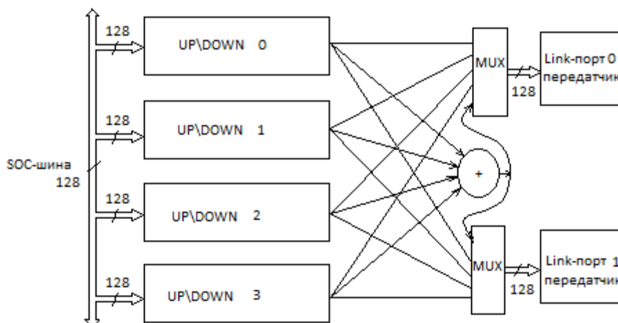
Рисунок 113 – Подключение модуля в режиме UP
