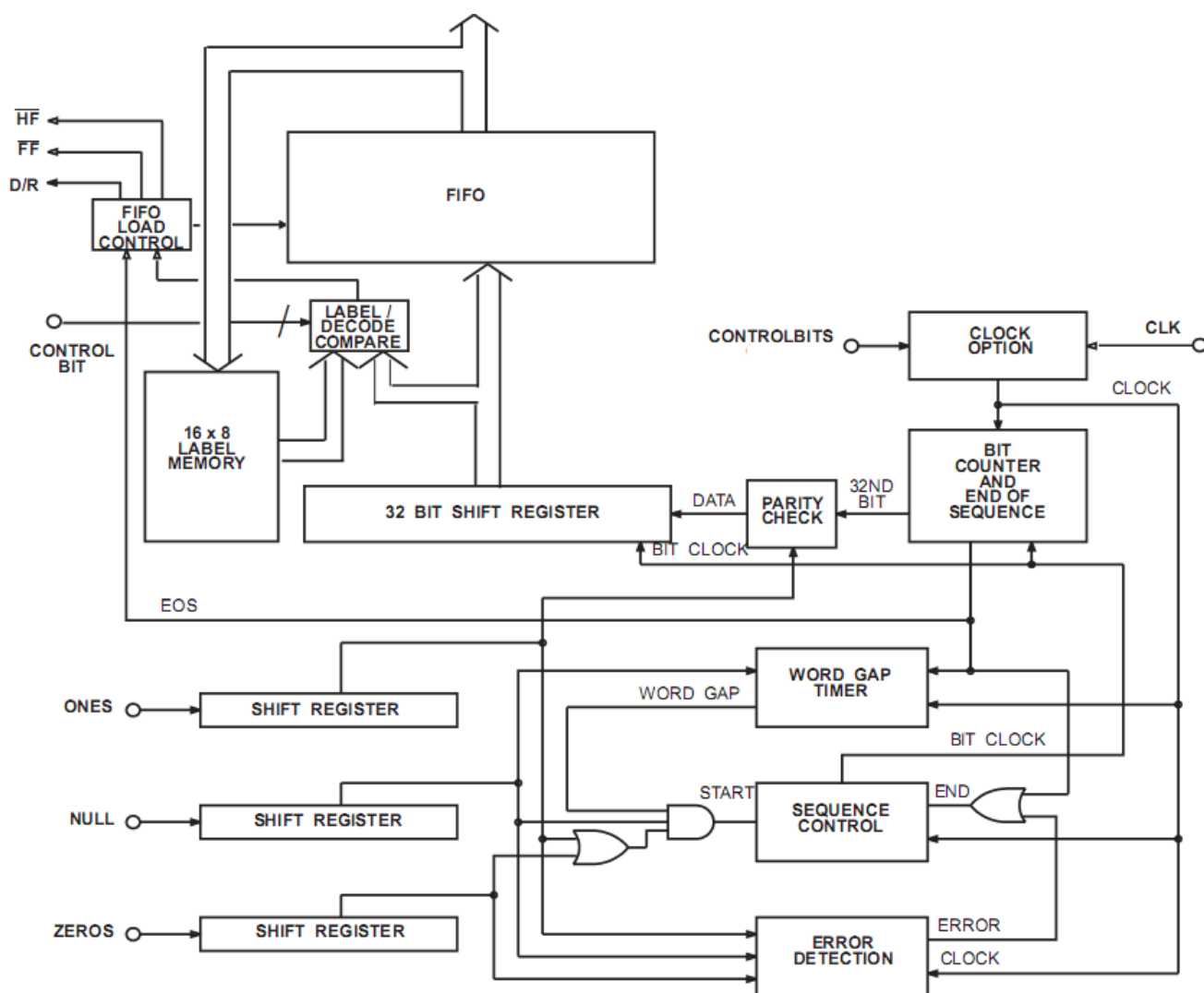
Рисунок 100 – Структурная схема канала приема
