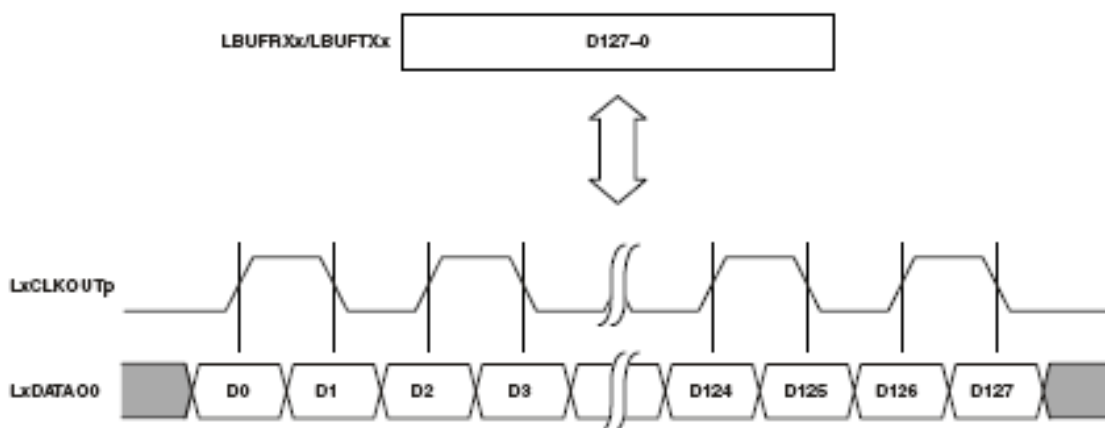
Рисунок 75 – Шина данных 1 разряд
