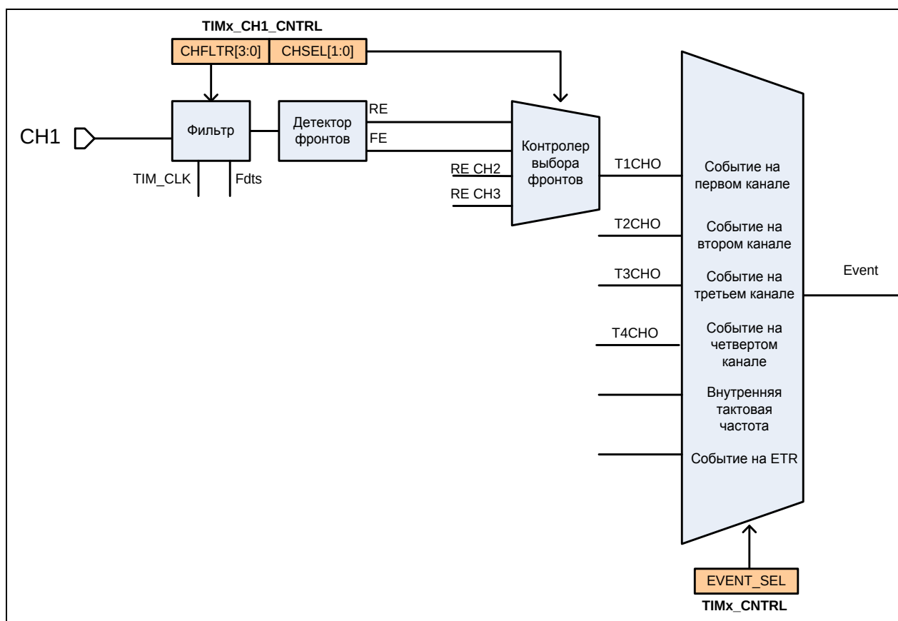
Рисунок 31 – Тактирование с входа первого канала
