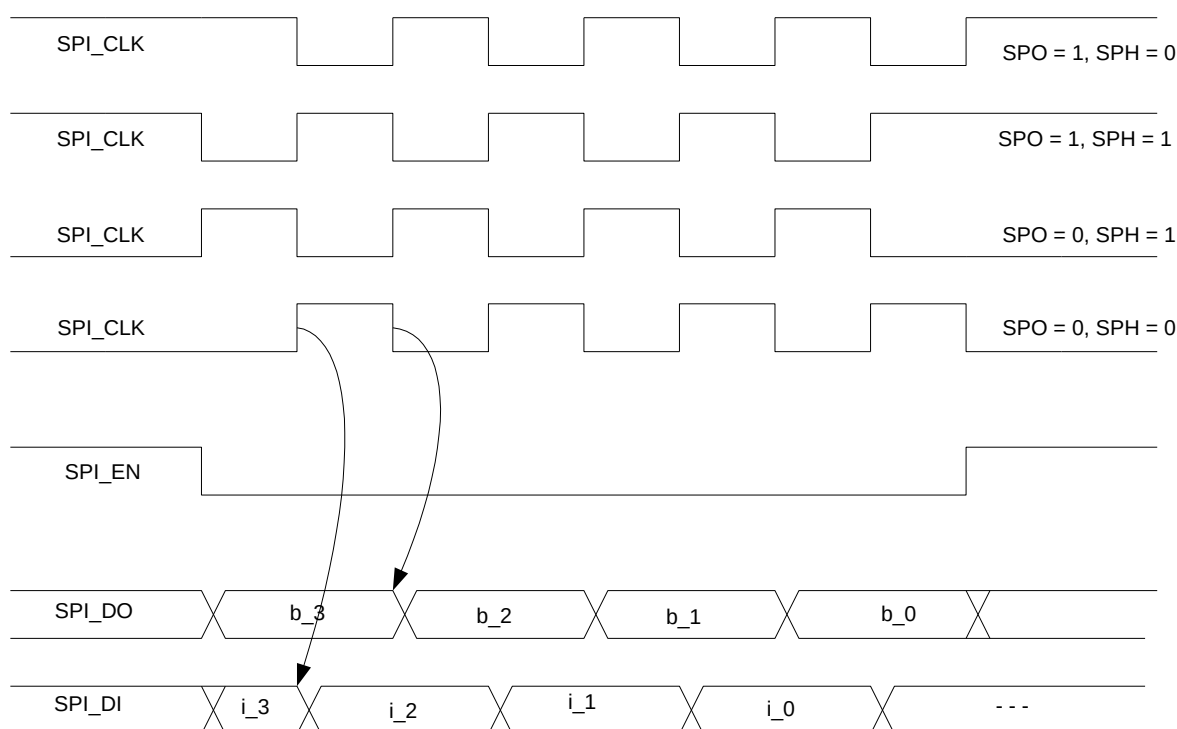
Рисунок 83 – Диаграмма обмена в режиме master
