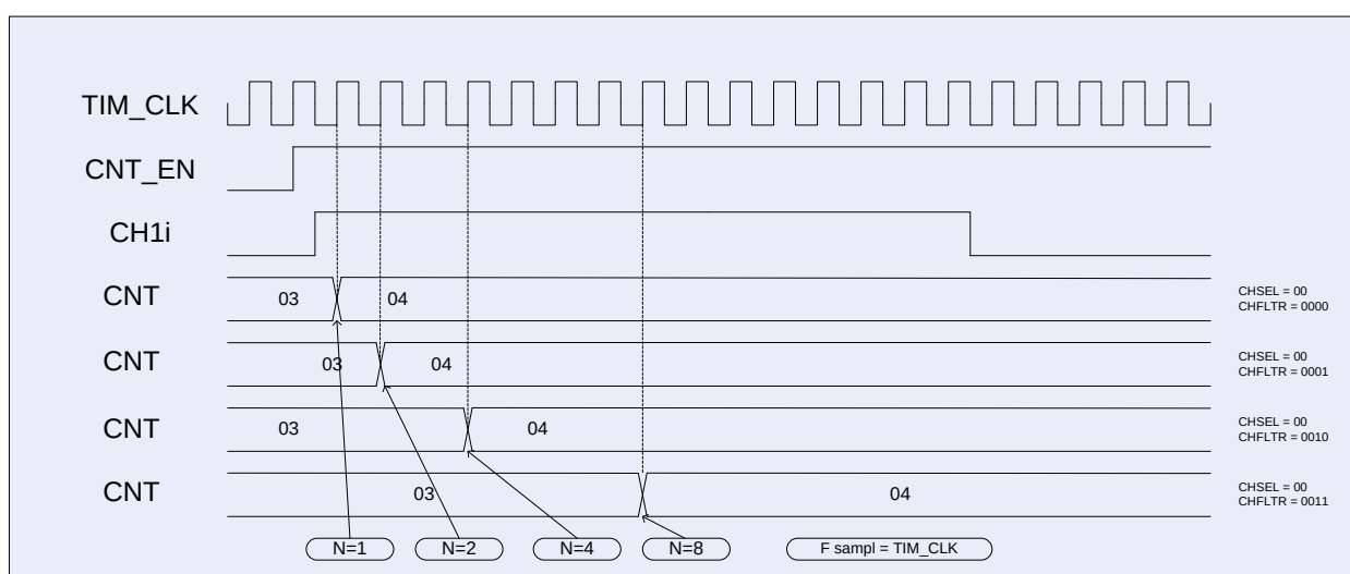
Рисунок 33 – Диаграмма внешнего тактирования с разными вариантами фильтра
