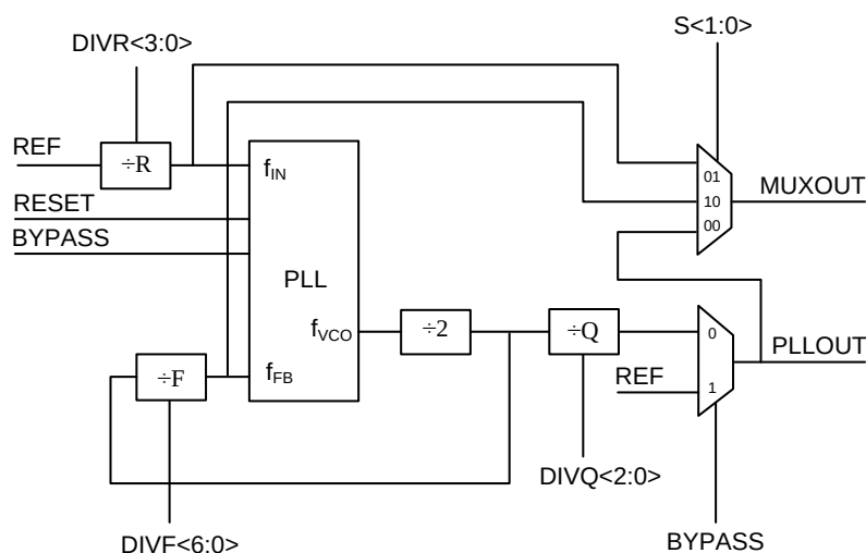
Рисунок 115 – Структура PLL
