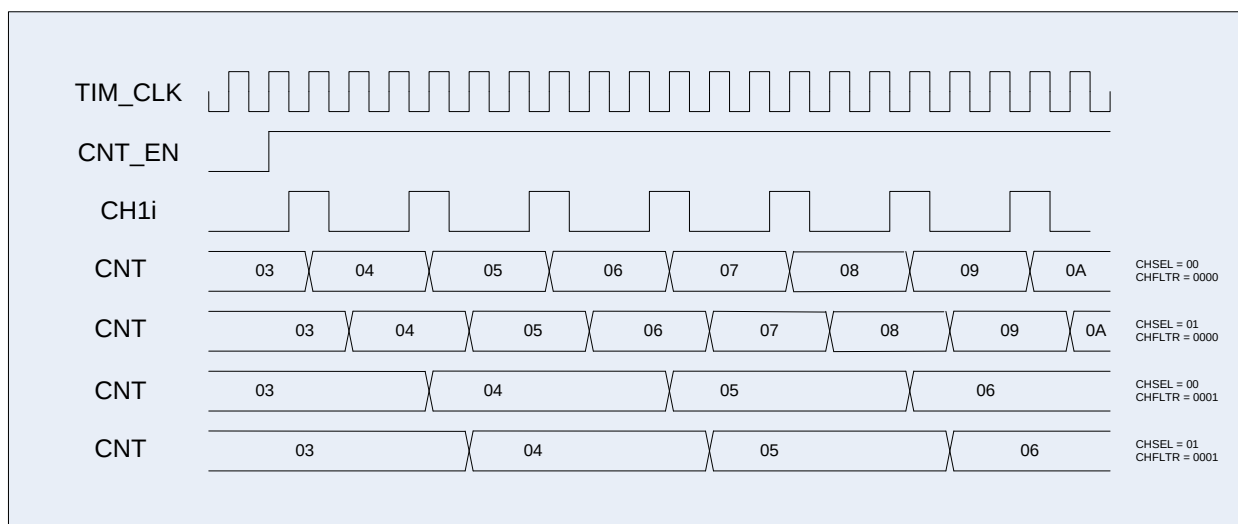
Рисунок 32 – Диаграмма внешнего тактирования с разными вариантами фильтра
