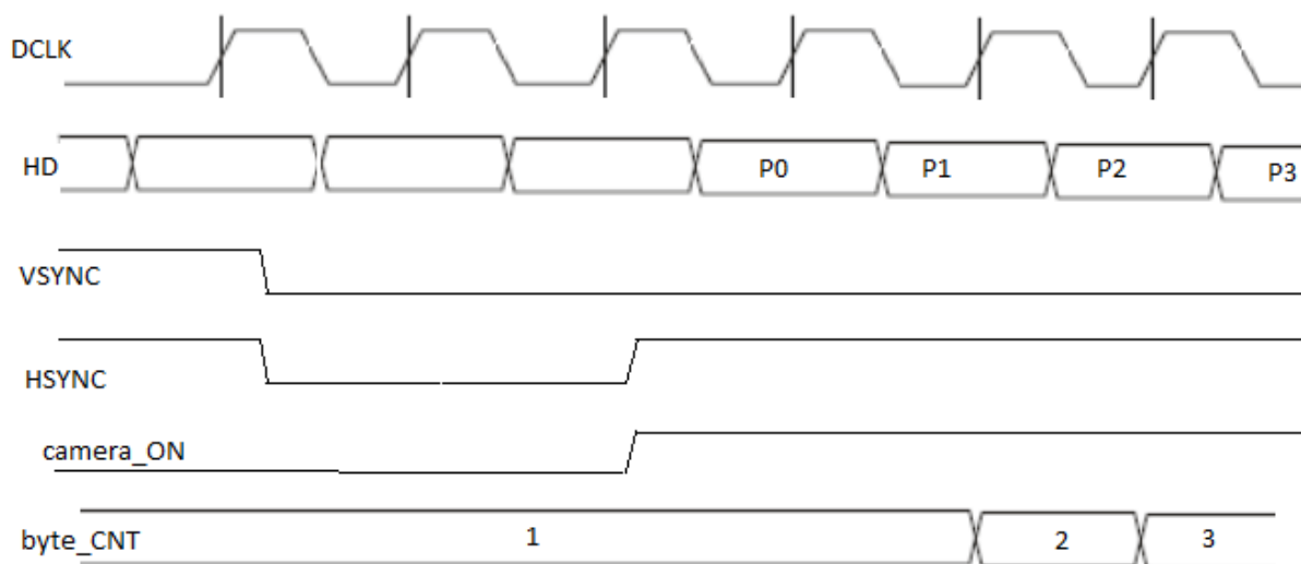
Рисунок 85 – Начало приема данных в режиме «видеокамера»
