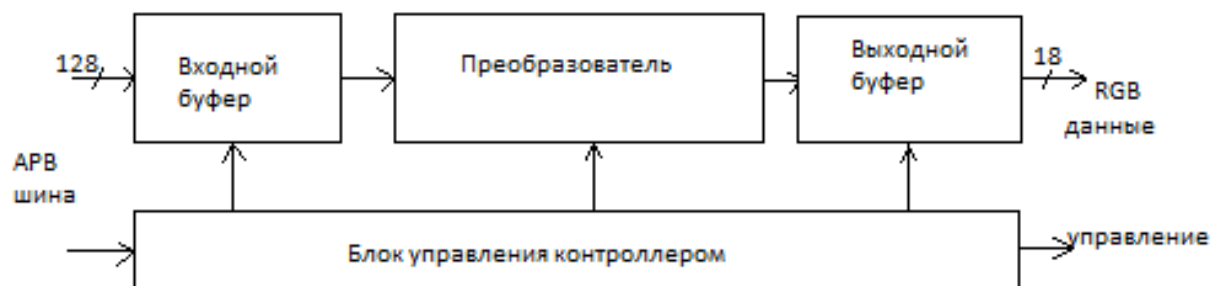
Рисунок 89 – Структура контроллера
