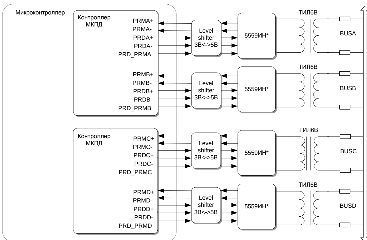
Рисунок 102 – Структурная схема контроллера интерфейса по ГОСТ Р 52070-2003
