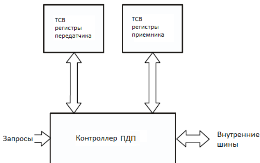
Рисунок 47 – Блок-схема DMA
