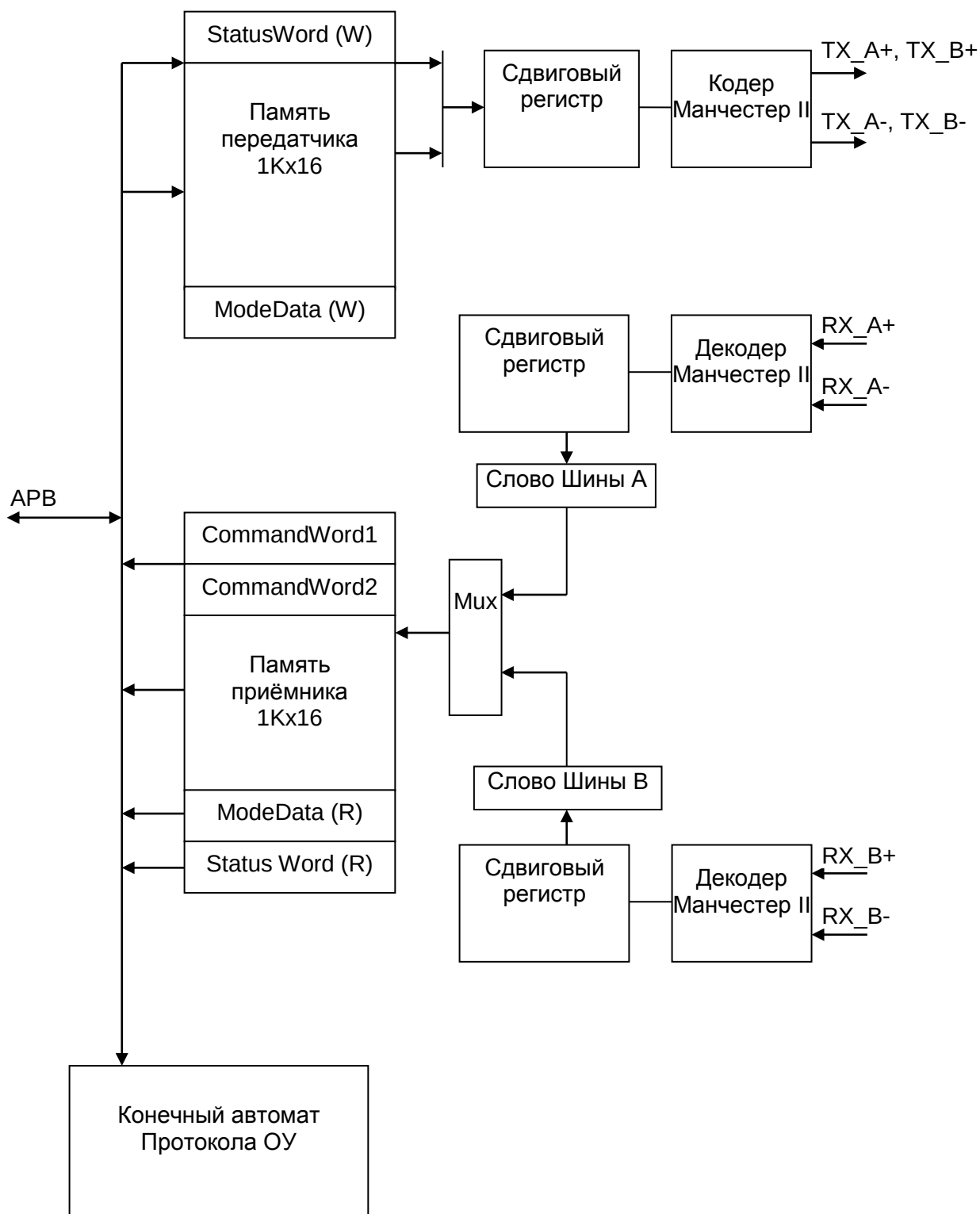
Рисунок 107 – Структурная схема работы в режиме ОУ
