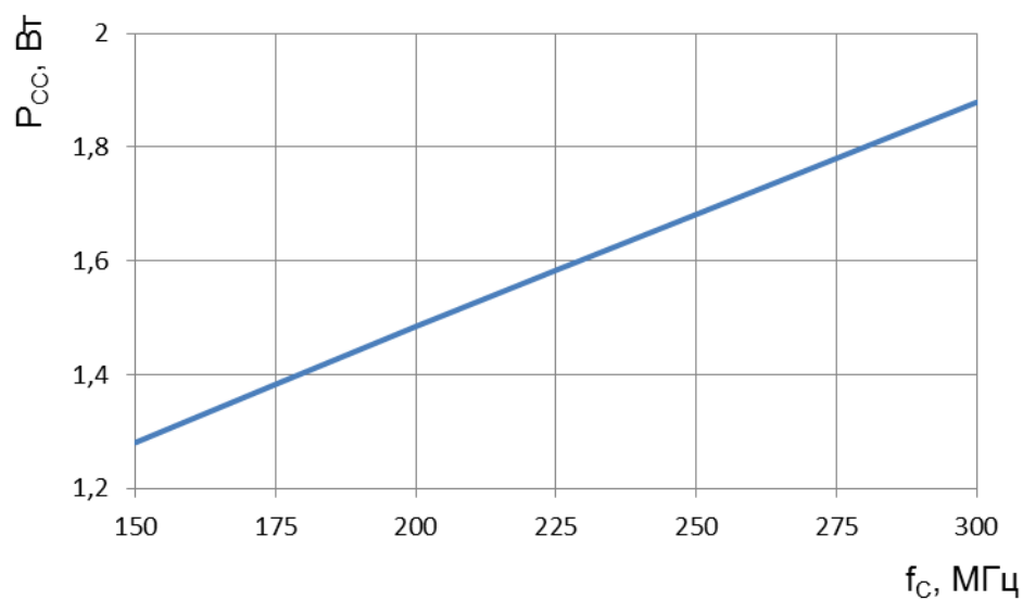
Рисунок 124 – Зависимость потребляемой мощности P_{cc} от тактовой частоты процессора f_c при U_{cc}= 1,32 В, U_{cca} = U_{ccio} = 3,6 В, f_{c\_PLL} = 50 МГц, T = 25 °С
