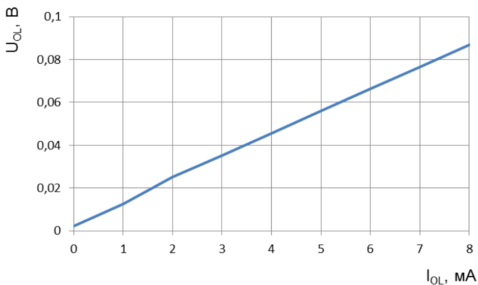
Рисунок 119 – Зависимость выходного напряжения низкого уровня U_{OL} от тока нагрузки при U_{CC} = 1,08 В, U_{CCA} = U_{CCIO} = 3,0 В, T = 25 °С
