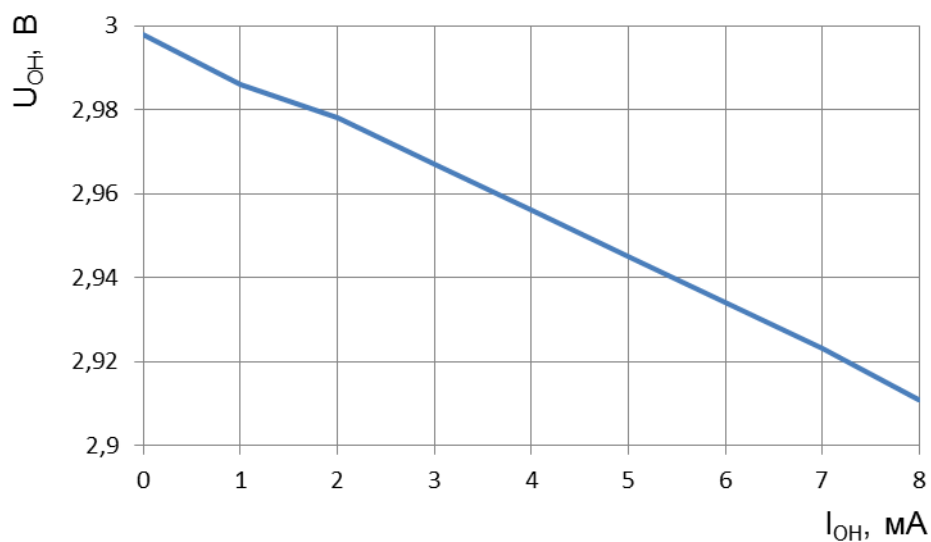
Рисунок 118 – Зависимость выходного напряжения высокого уровня U_{OH} от тока нагрузки при U_{CC} = 1,08 В, U_{CCA} = U_{CCIO} = 3,0 В, T = 25 °С
