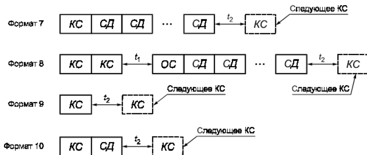
Рисунок 104 – Форматы групповых сообщений
