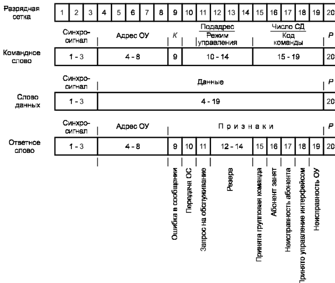
Рисунок 105 – Форматы слов
