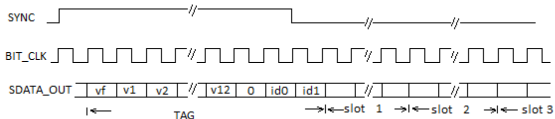
Рисунок 93 – Структура тега
