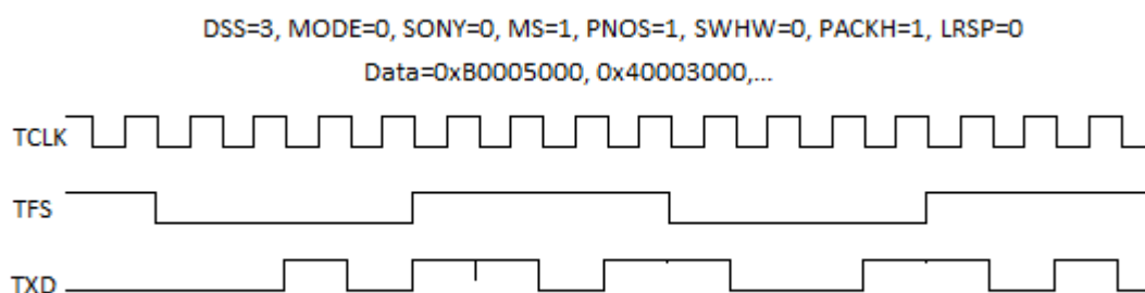
Рисунок 95 – Выдача информации по отрицательному фронту TCLK
