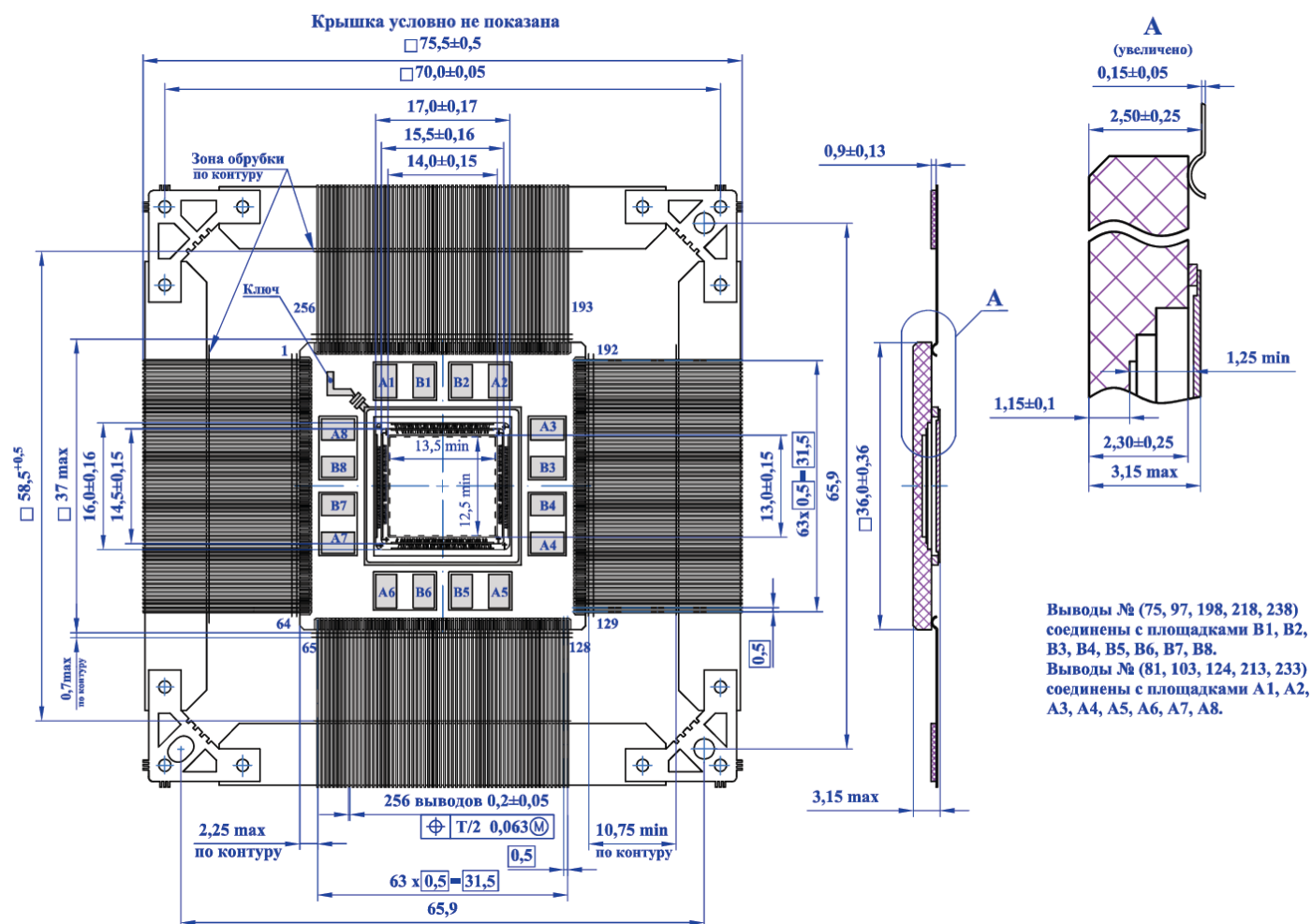
Рисунок 125 – Микросхема в корпусе 4244.256-3
