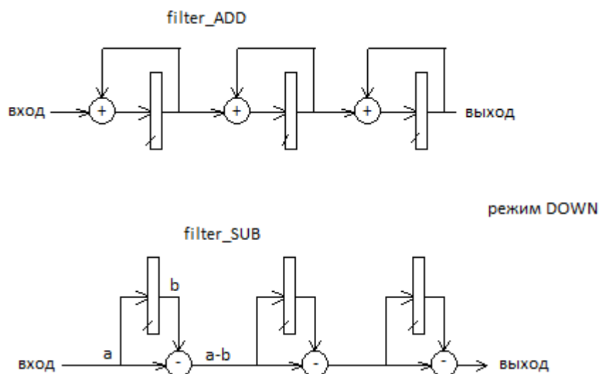
Рисунок 110 – Структура фильтров для режима DOWN
