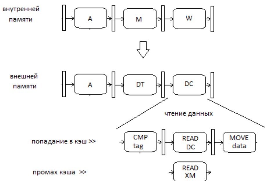
Рисунок 14 – Конвейер обработки данных
