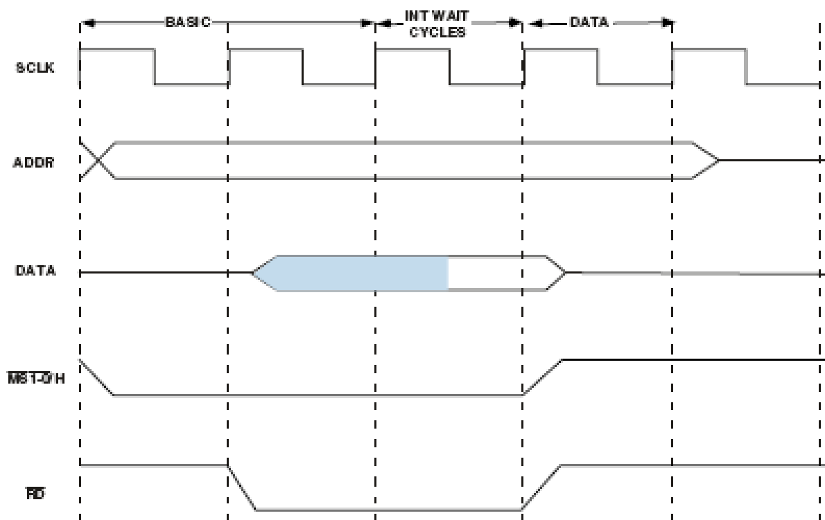
Рисунок 59 – Медленный протокол. Чтение с циклами ожидания
