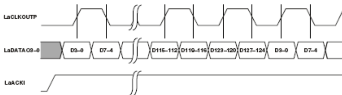
Рисунок 76 – Порт связи “а” передает слова порту связи “b” одно за другим
