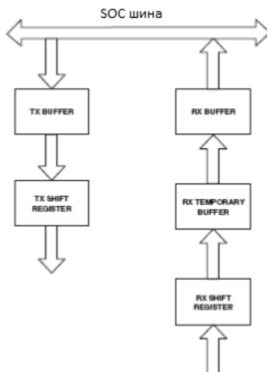
Рисунок 69 – Архитектура порта связи
