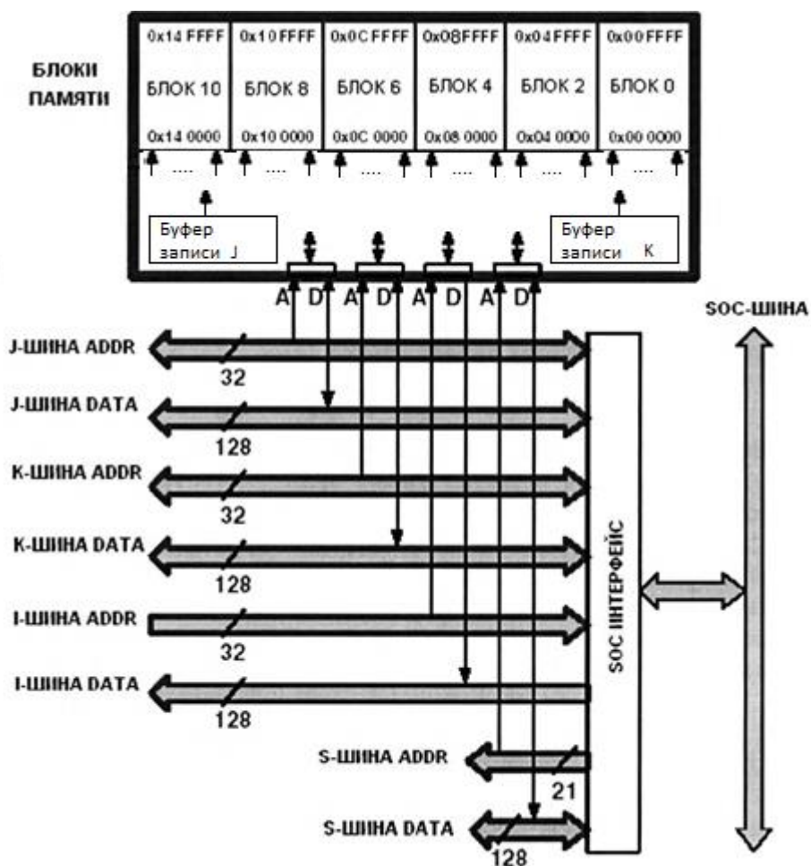
Рисунок 4 – Подключение внутренней памяти к ядру процессора
