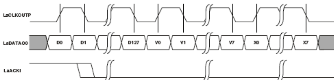
Рисунок 78 – Порт связи “а” передает порту связи “b” с верификацией
