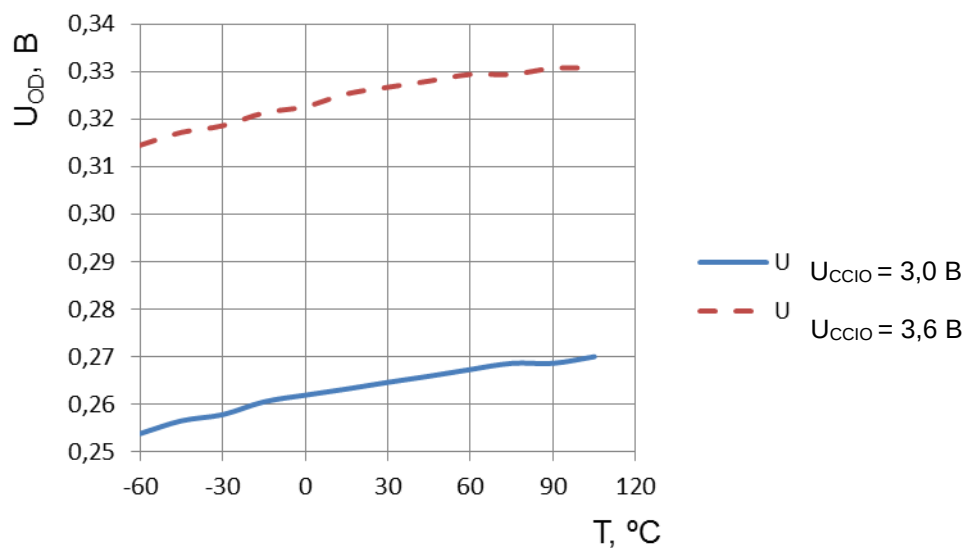
Рисунок 120 – Зависимость дифференциального выходного напряжения LINK-портов U_{OB} от температуры при R_L=100 \text{ Ом}
