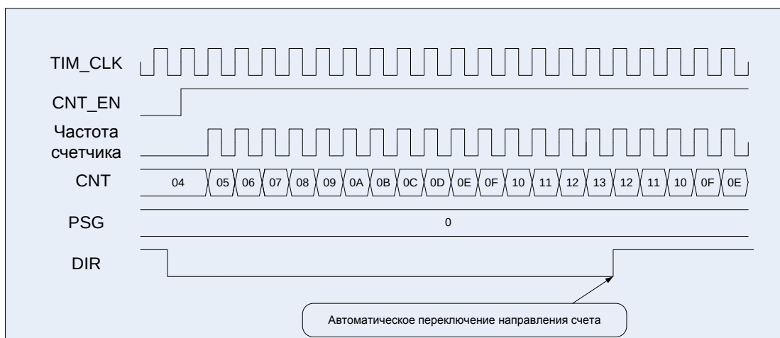
Рисунок 22 – Диаграммы работы таймера, счет вверх/вниз, сначала вверх
