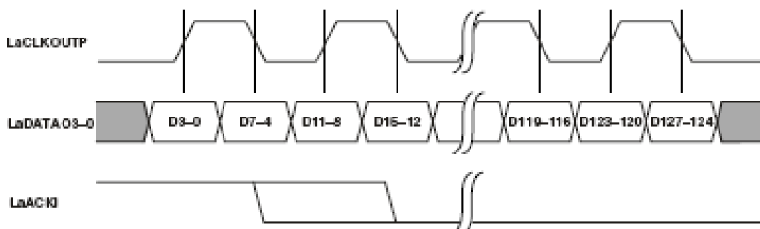
Рисунок 77 – Порт связи “а” передает порту связи “b” (приемник заполнен)
