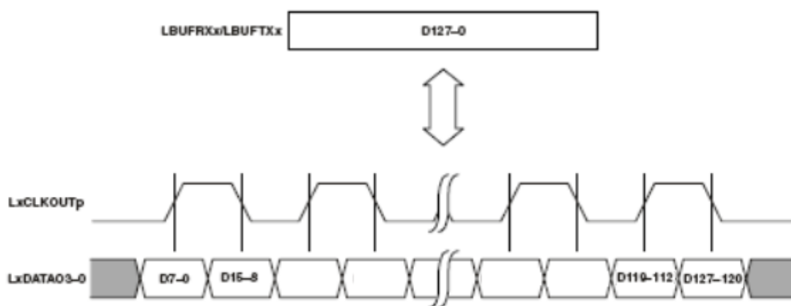
Рисунок 73 – Шина данных 8 разрядов
