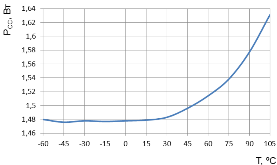
Рисунок 122 – Зависимость потребляемой мощности P_{CC} от температуры при U_{CC} = 1,32 В, U_{CCA} = U_{CCIO} = 3,6 В, f_C = 230 МГц, f_{C\_PLL} = 50 МГц
