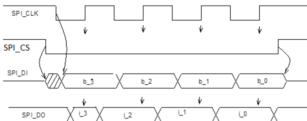
Рисунок 84 – Диаграмма обмена в режиме slave
