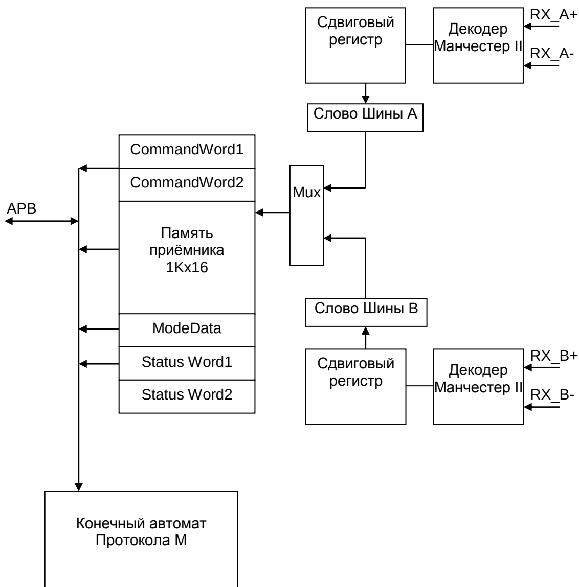
Рисунок 108 – Структурная схема работы в режиме M
