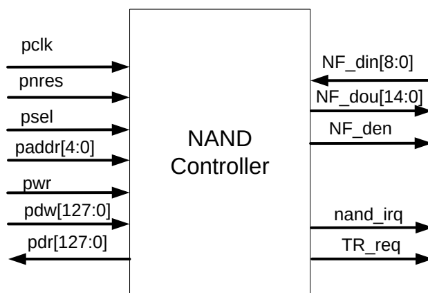
Рисунок 87 – Условное графическое обозначение контроллера
