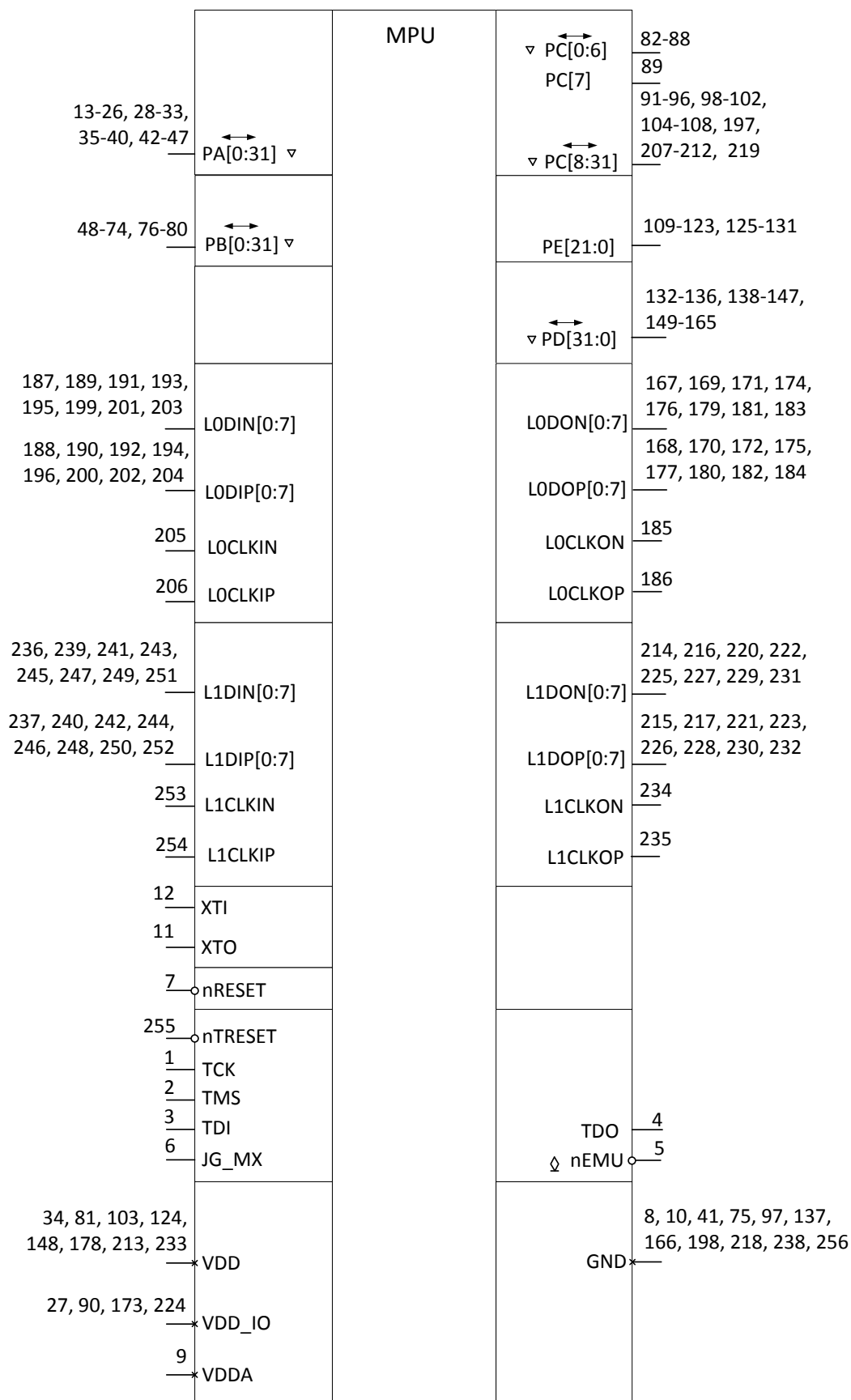
Рисунок 2 – Условно-графическое обозначение
