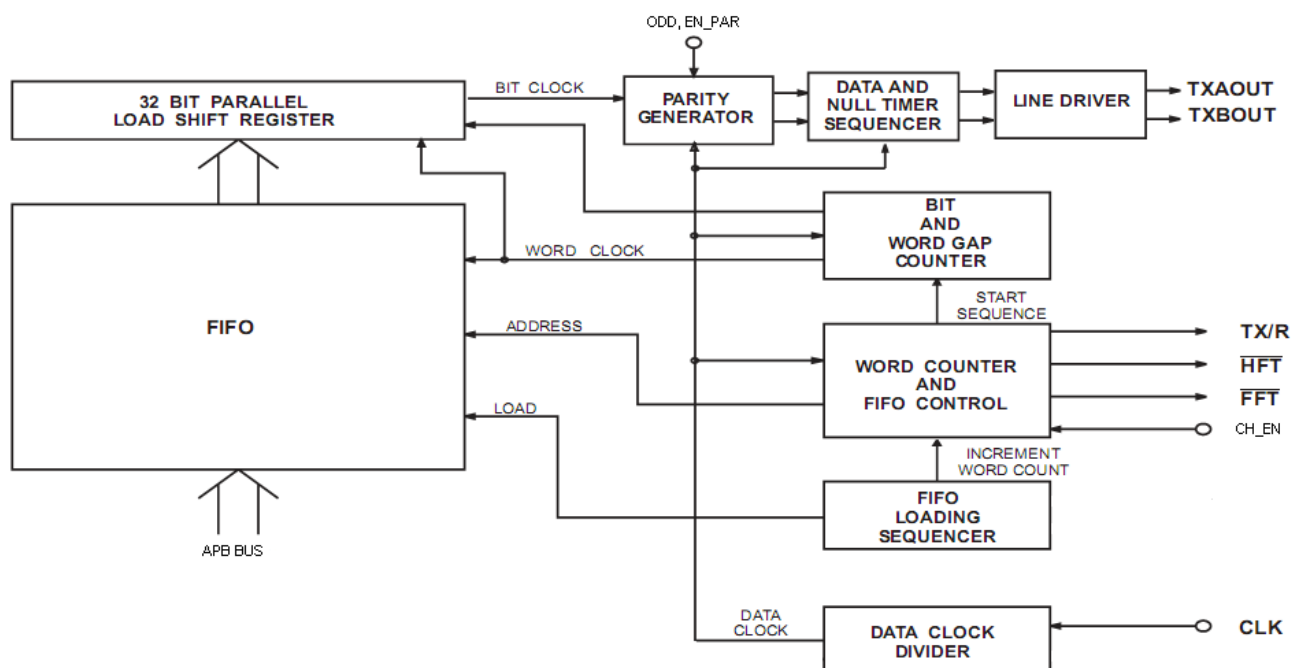
Рисунок 101 – Структурная схема канала передачи
