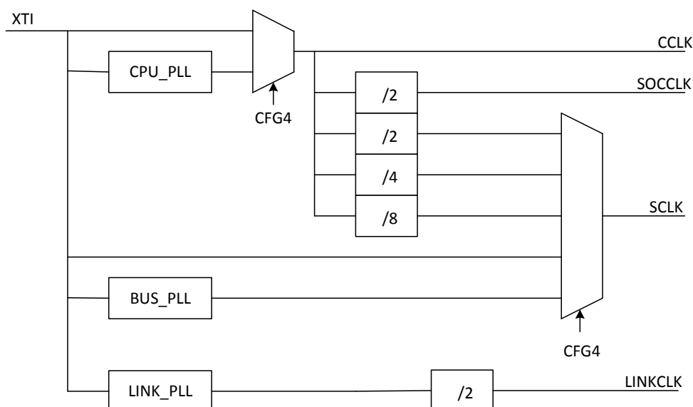
Рисунок 114 – Источники тактовой частоты
