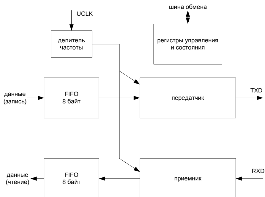
Рисунок 82 – Структурная схема UART
