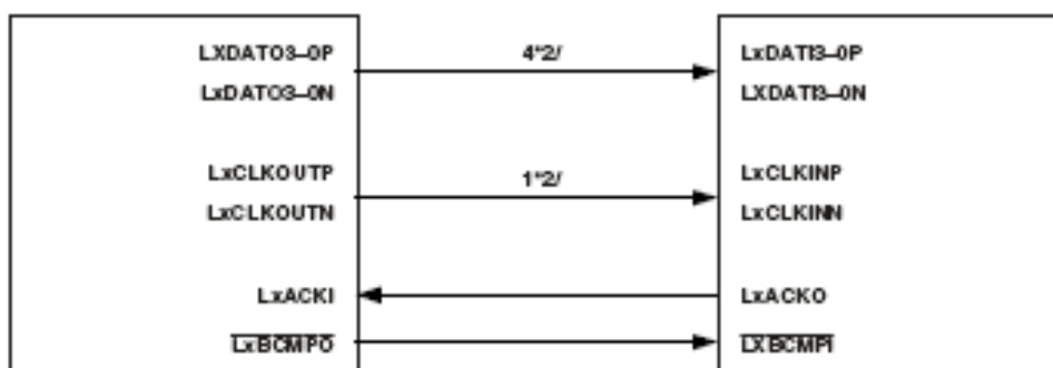
Рисунок 70 – Конфигурация порта связи (4-разрядный режим)
