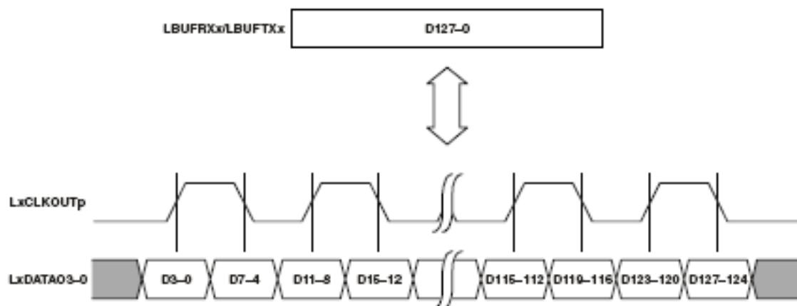
Рисунок 74 – Шина данных 4 разряда
