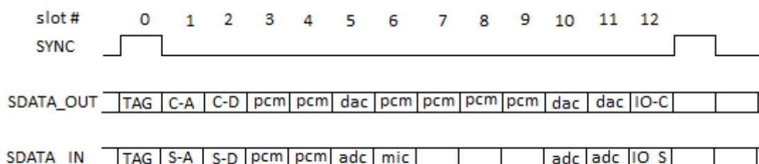
Рисунок 92 – Структура фрейма
