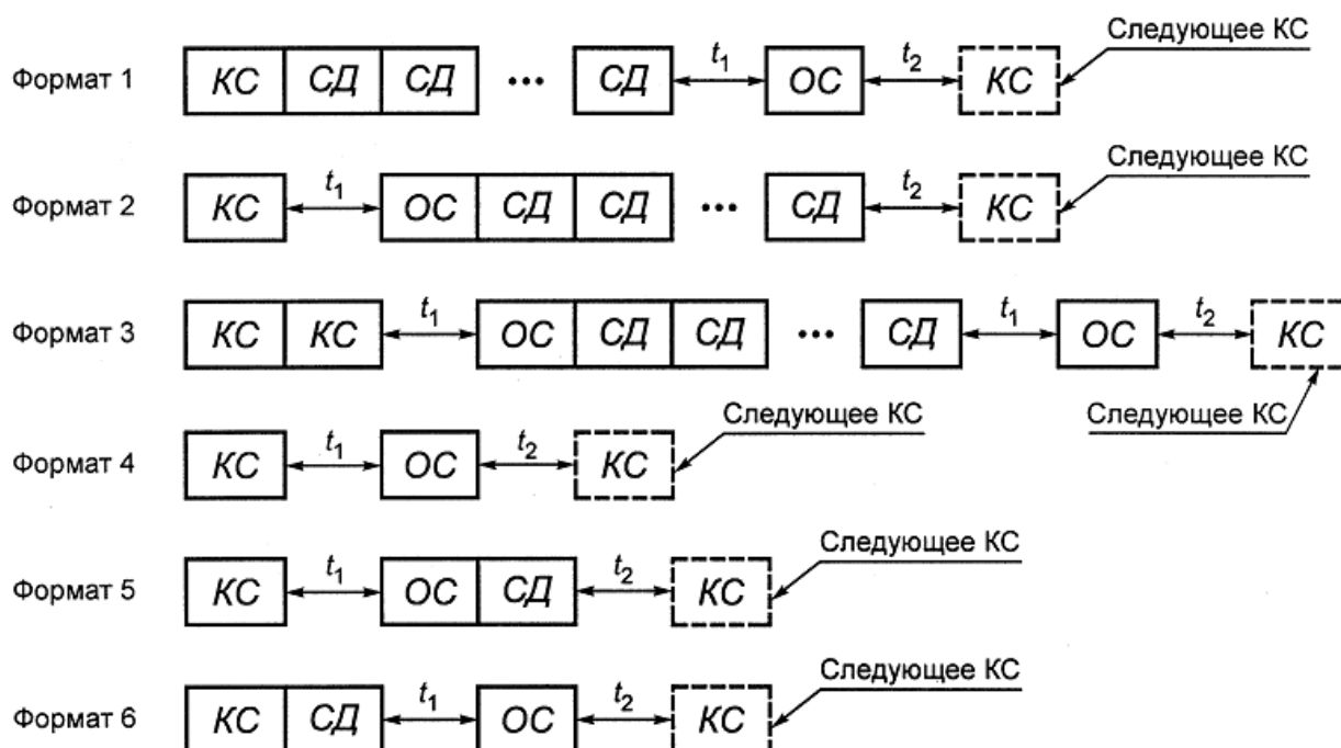
Рисунок 103 – Форматы сообщений
