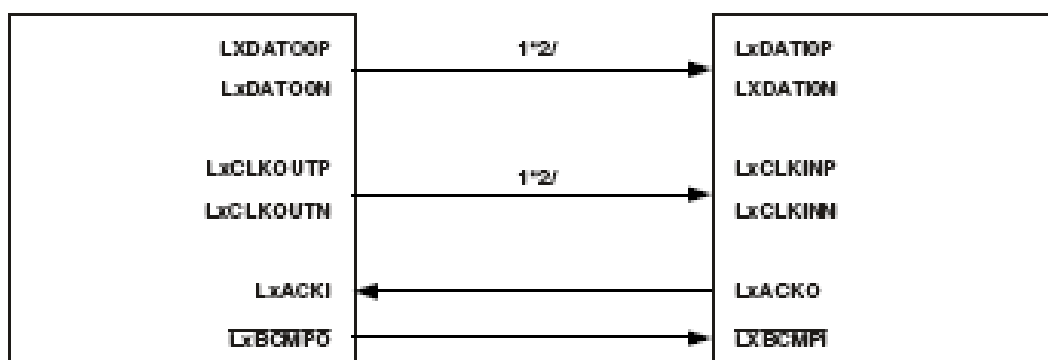
Рисунок 71 – Конфигурация порта связи (1-разрядный режим)
