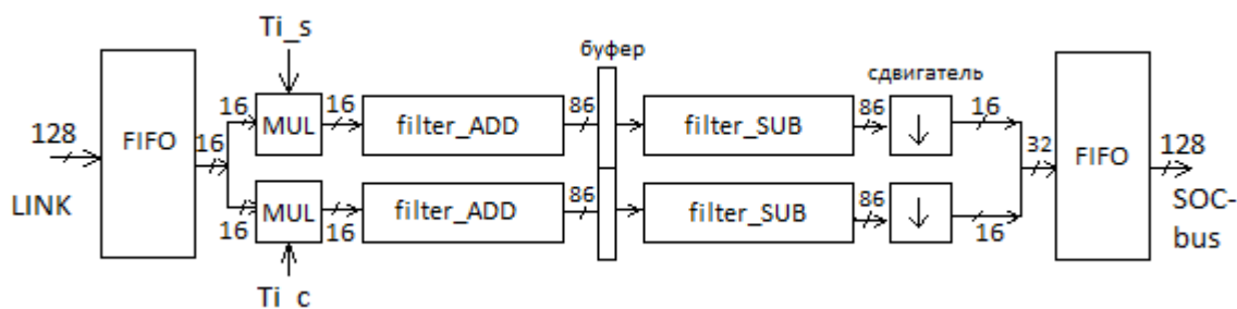
Рисунок 109 – Структура модуля в режиме DOWN
