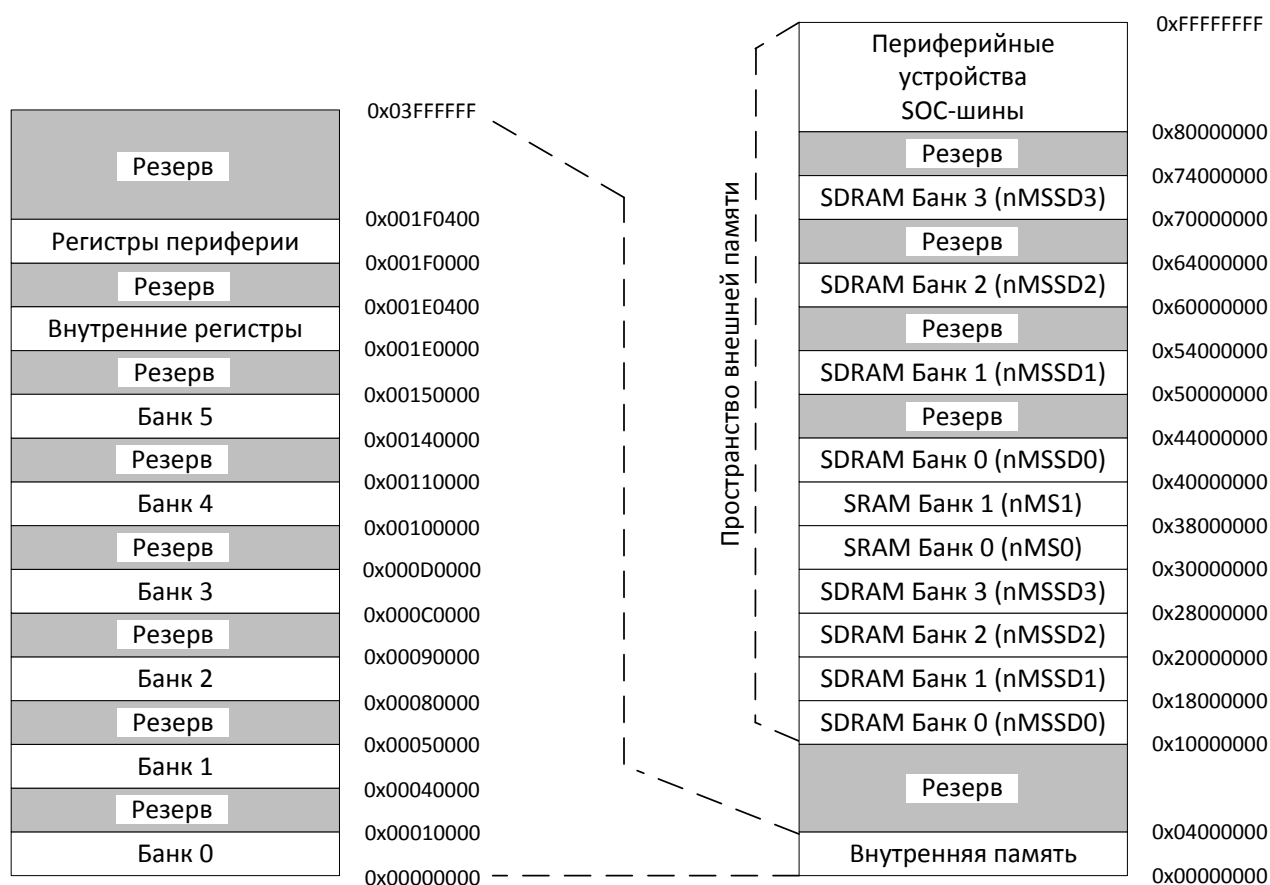
Рисунок 9 – Карта памяти (байтовая адресация)
