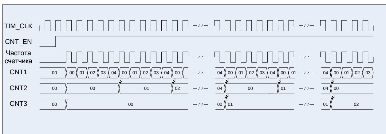
Рисунок 29 – Диаграммы работы трех таймеров в каскаде
