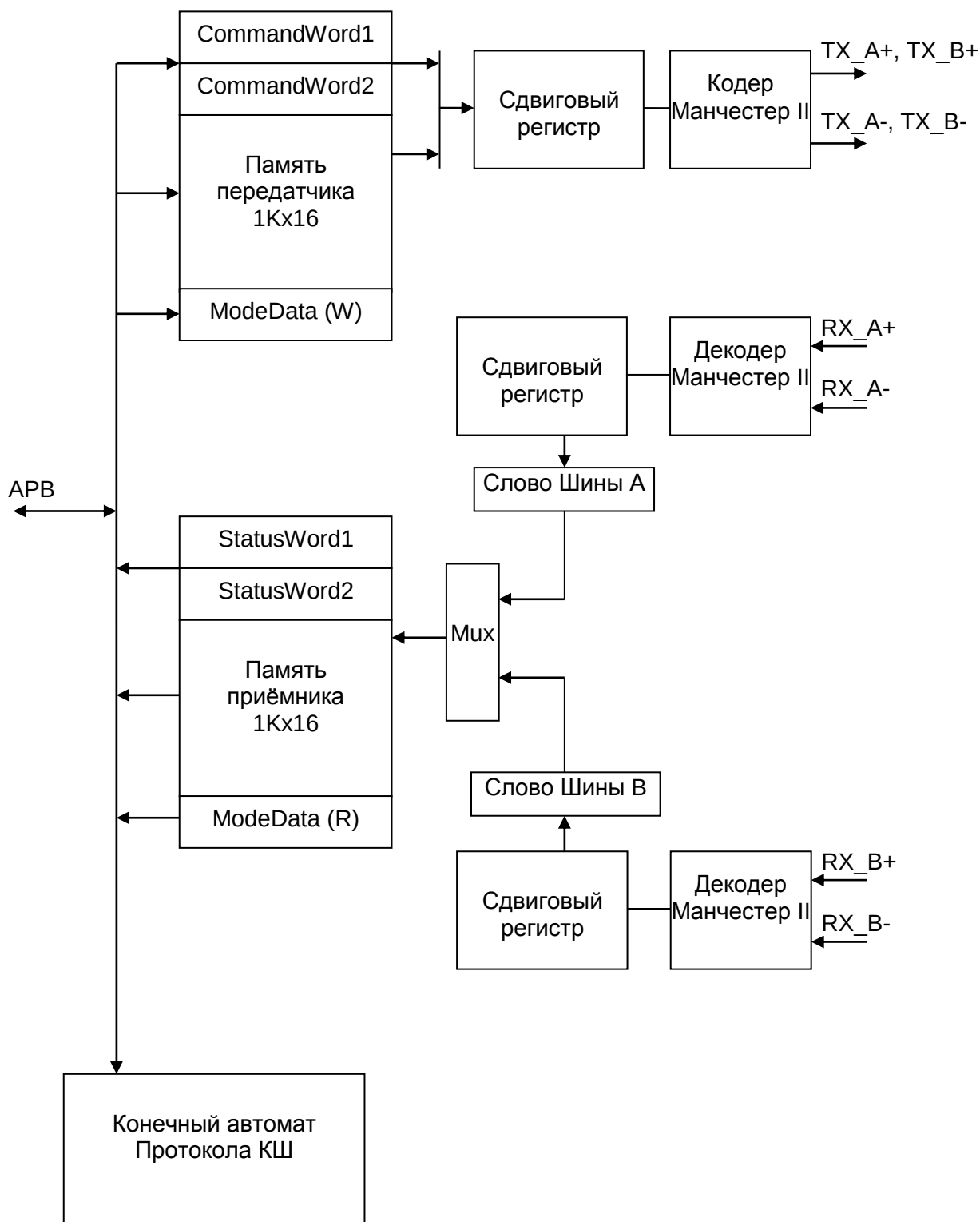
Рисунок 106 – Структурная схема работы в режиме КШ
