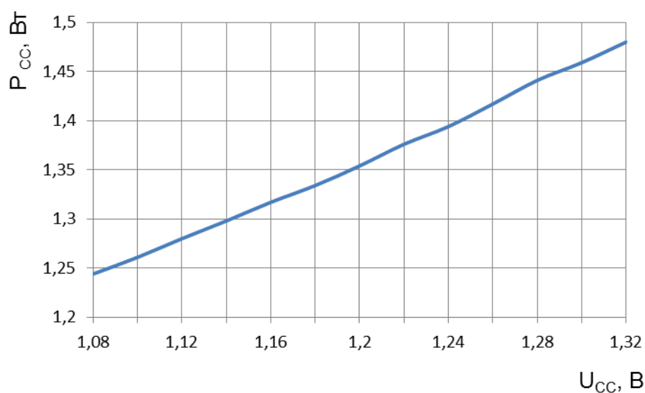
Рисунок 123 – Зависимость потребляемой мощности P_{CC} от напряжения питания ядра U_{CC} при U_{CCA} = U_{CCIO} = 3,6 В, f_C = 230 МГц, f_{C\_PLL} = 50 МГц, T = 25 °C
