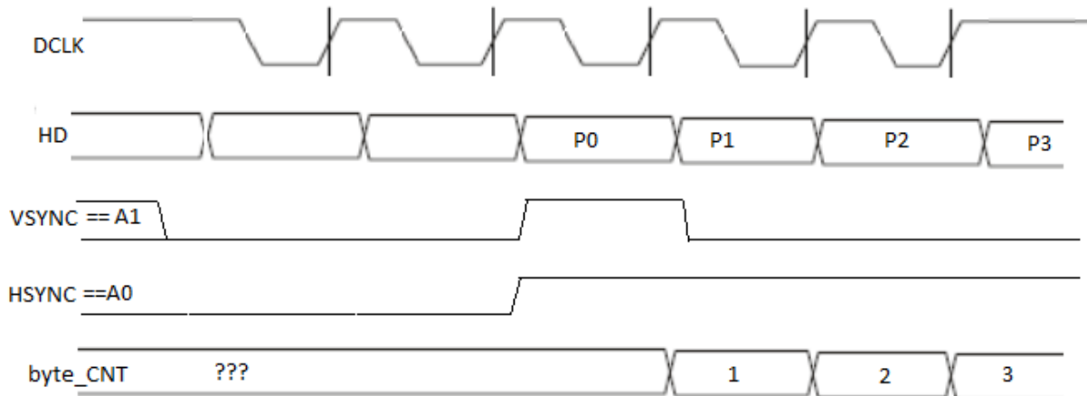
Рисунок 86 – Начало приема данных в режиме «ведущее устройство»
