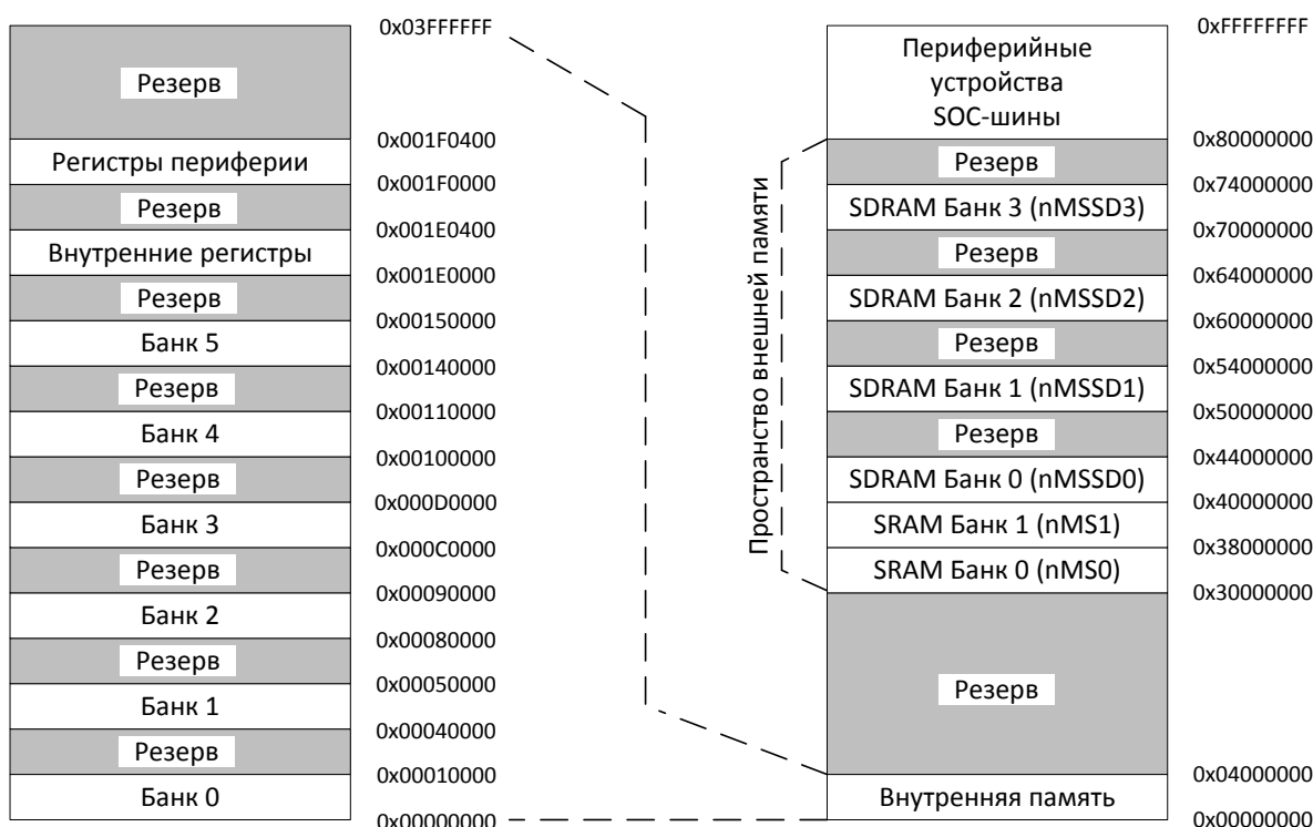
Рисунок 8 – Базовая карта памяти (словная адресация)
