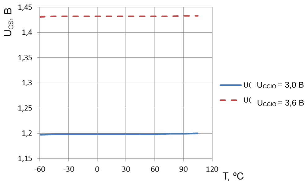
Рисунок 121 – Зависимость синфазного выходного напряжения LINK портов U_{Os} от температуры при R_L=100 \text{ Ом}
