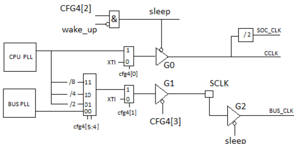
Рисунок 116 – Схема блокировки синхронизации
