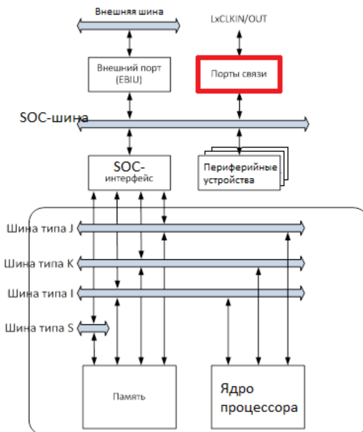
Рисунок 68 – Подключение портов связи на кристалле
