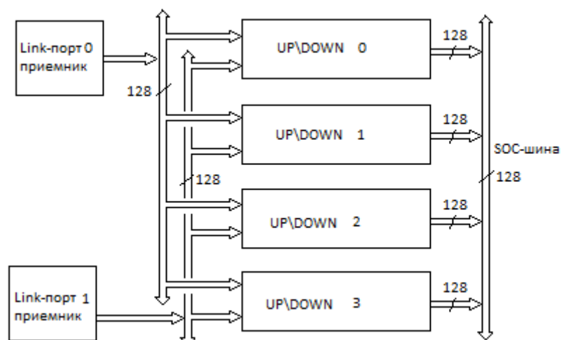
Рисунок 112 – Подключение модуля в режиме DOWN
