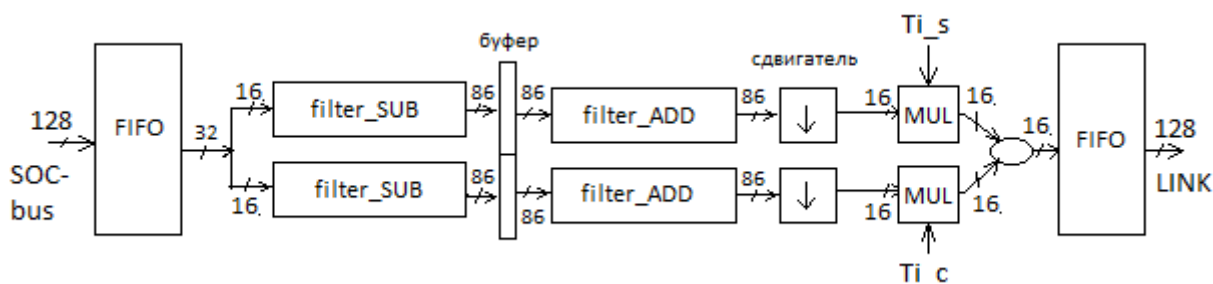
Рисунок 111 – Структура модуля в режиме UP
