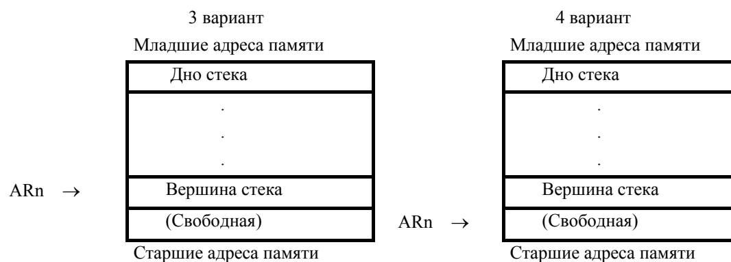
Рисунок 5.31 - Реализация стеков от младших адресов памяти к старшим
