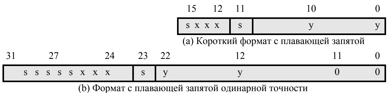
Рисунок 4.9 - Преобразование короткого формата с плавающей запятой в формат с плавающей запятой одинарной точности
