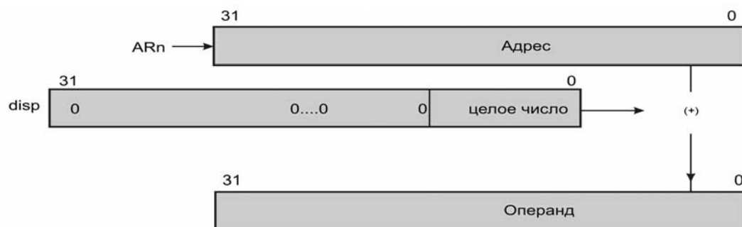
Рисунок 5.3 - Косвенная адресация с предварительным добавлением смещения
