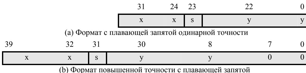
Рисунок 4.11 - Преобразование формата с плавающей запятой одинарной точности в формат с плавающей запятой повышенной точности
