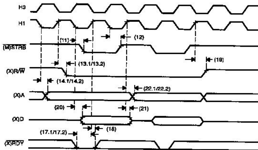
Рисунок 11.23 - Временные диаграммы записи памяти ( \overline{(M)STRB} = 0 )
