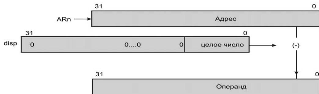
Рисунок 5.4 - Косвенная адресация с предварительным вычитанием смещения
