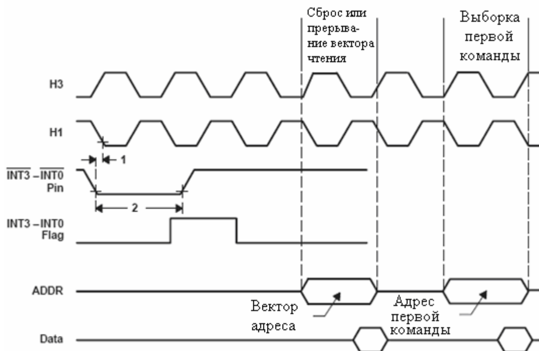
Рисунок 11.35 - Временные диаграммы отклика на \overline{INT3-INT0}
