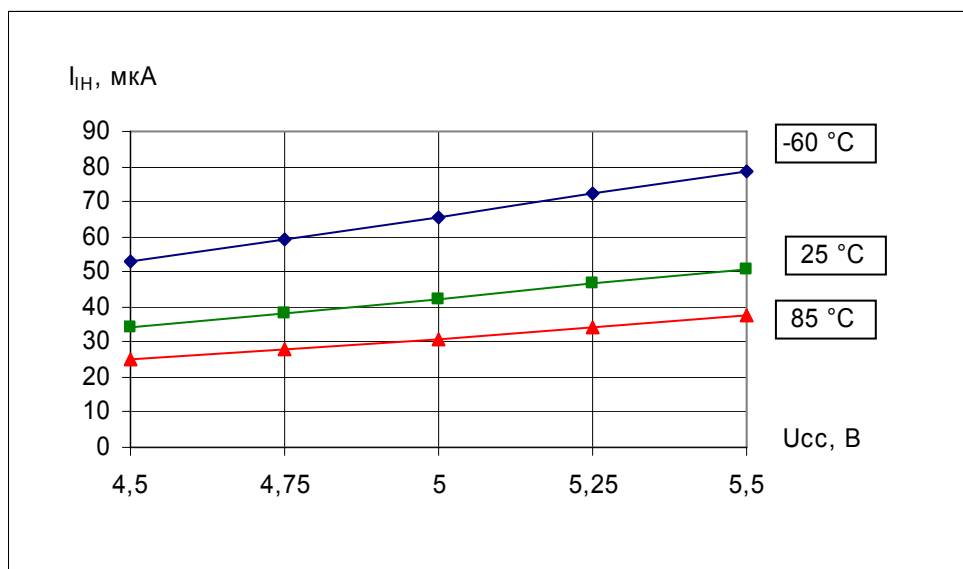
Рисунок 11.10 - Зависимость входного тока высокого уровня I_{IN} по входу X2/CLKIN от напряжения питания U_{CC} при U_I=U_{CC} (норма не более 90\text{ мкА} )
