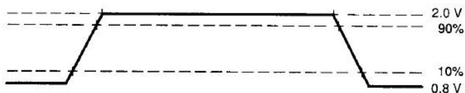
Рисунок 11.19 - Входы с ТТЛ-уровнем
