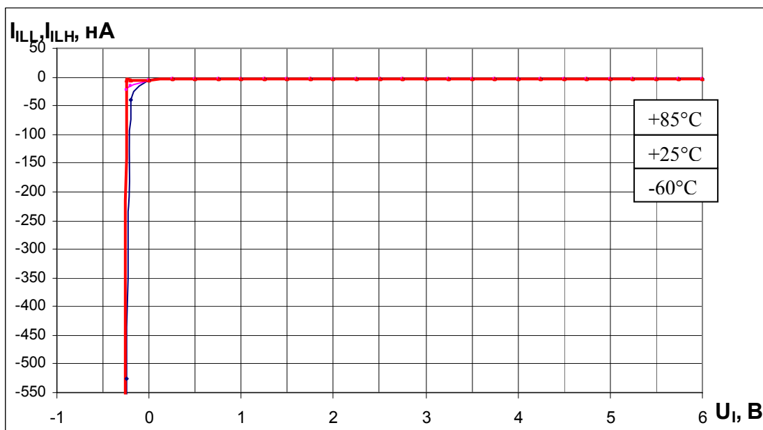
Рисунок 11.7 - Зависимость тока утечки I_{ILL}, I_{ILH} входов типа \overline{RDY}, \overline{HOLD} от входного напряжения U_I при U_{CC}=5,5 В (при U_I = -0,5 В I_{ILL} = -5 мкА при температуре 85 °С, I_{ILL} = -7,1 мкА при температуре 25 °С, I_{ILL} = -8,2 мкА при температуре – 60 °С) (норма не менее -10 мкА, не более 10 мкА)
