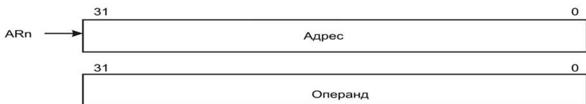
Рисунок 5.2 - Косвенная адресация через вспомогательный регистр
