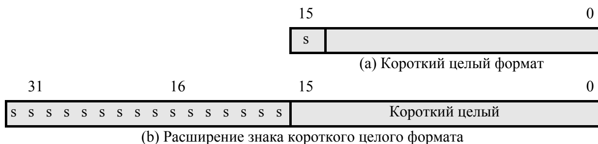
Рисунок 4.1 - Короткий целый формат и расширение знака короткого целого
