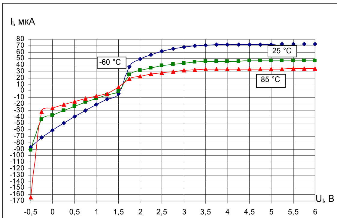
Рисунок 11.9 - Зависимость входного тока I_I по входу X2/CLKIN от входного напряжения U_I при U_{CC}=5,5\text{ В} (норма не менее -90\text{ мкА} , не более 90\text{ мкА} )
