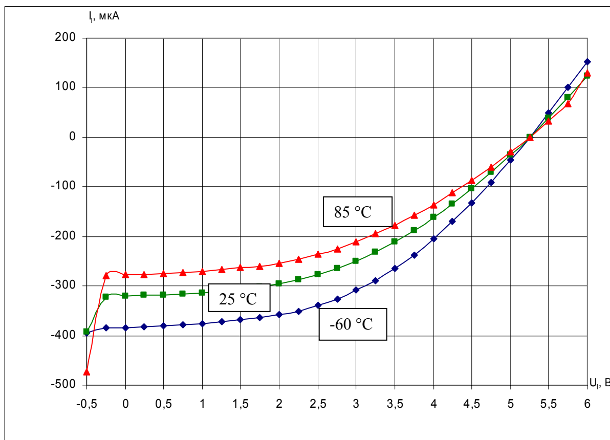
Рисунок 11.8 - Зависимость входного тока I_I входов \overline{INT0} - \overline{INT3}, \overline{RSV0} - \overline{RSV4}, \overline{MC} / \overline{MP} от входного напряжения U_I при U_{CC}=5,5 В (норма не менее -600 мкА, не более 20 мкА)
