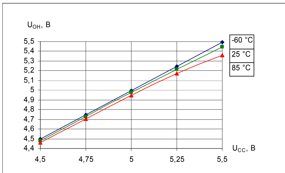
Рисунок 11.5 - Зависимость выходного напряжения высокого уровня U_{OH} от напряжения питания U_{CC} , при I_{OH} = -0,3\text{ mA} (норма не менее 2,4 В)
