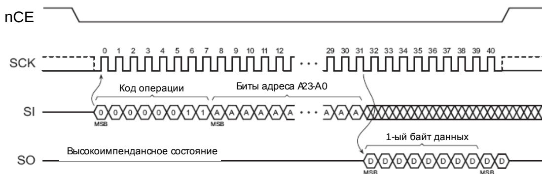
Рисунок 15 – Операция чтения с кодом 03h
