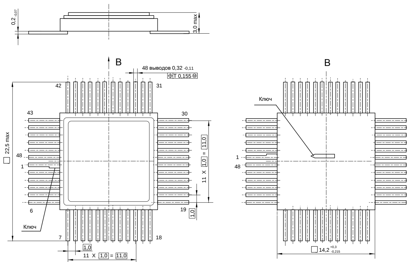
Рисунок 37 – Микросхема в корпусе Н16.48-1В
