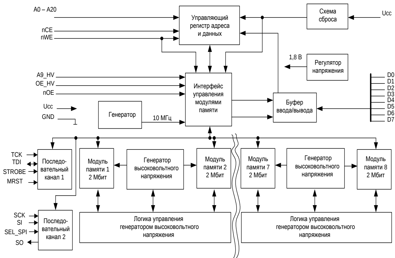
Рисунок 1 – Структурная блок-схема микросхемы
