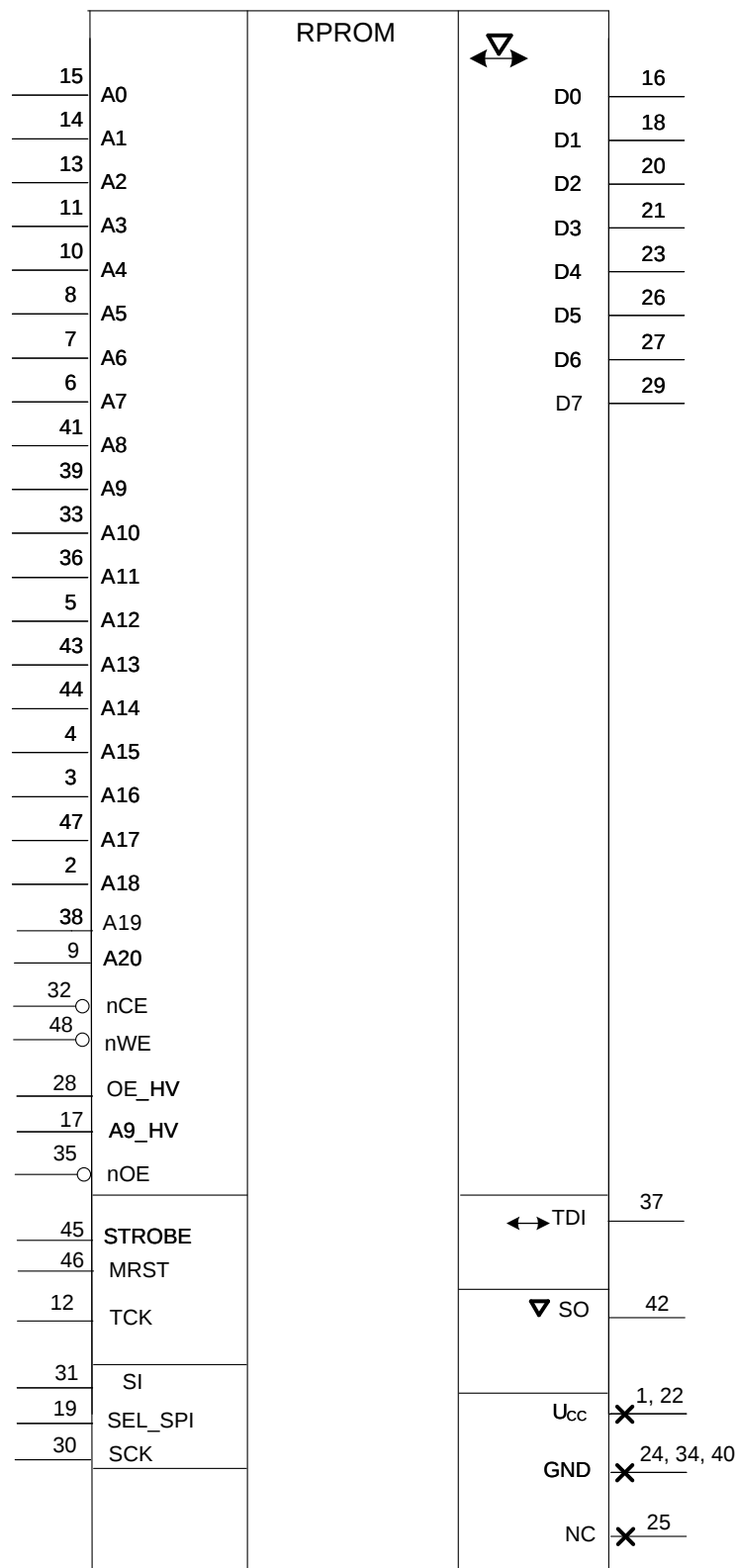
Рисунок 2 – Условно-графическое обозначение
