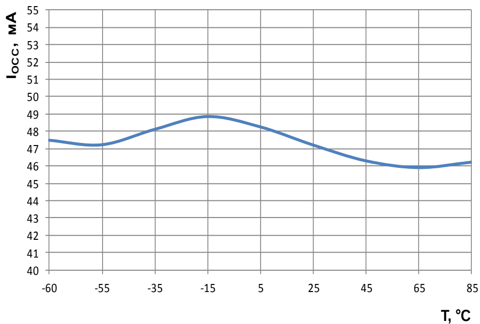
Рисунок 6 – Зависимость динамического тока потребления ( I_{osc} ) от температуры при R_L = 45 Ом на выходах CANH, CANL, напряжении питания 5,5 В
