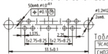
Рисунок 21 соединителей СМП268-15
