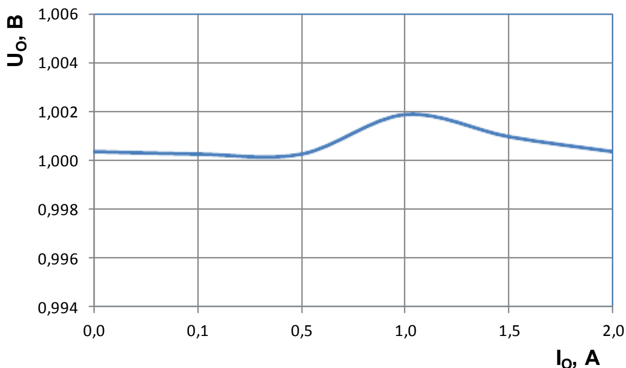
Рисунок 10 – Зависимость минимального выходного напряжения U_o микросхемы 1309EP1T от тока нагрузки при U_i = 2,5 В, T = 25 °C
