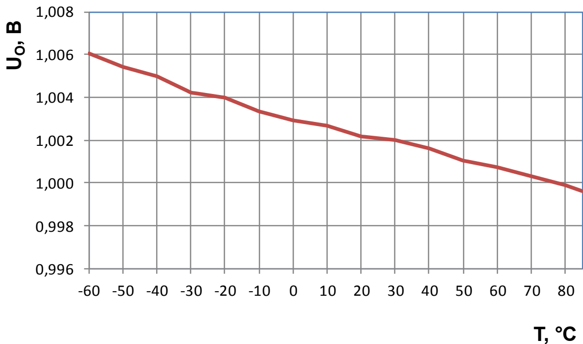
Рисунок 6 – Зависимость минимального выходного напряжения U_o микросхемы 1309ЕР1Т от температуры корпуса при U_i = 2 В, I_o = 10 мА
