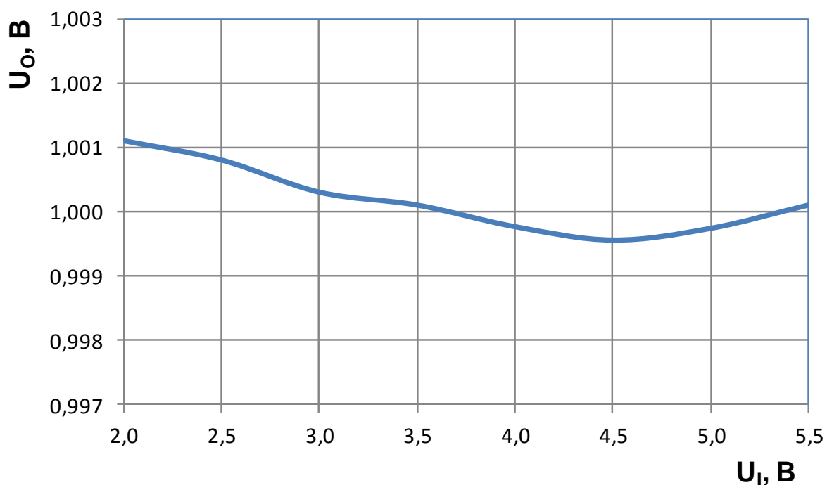
Рисунок 8 – Зависимость минимального выходного напряжения U_o микросхемы 1309ЕР1Т от входного напряжения при I_o = 100 мА, T = 25 °С
