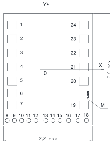
Рисунок 20 – Корпус 4116.8-3
