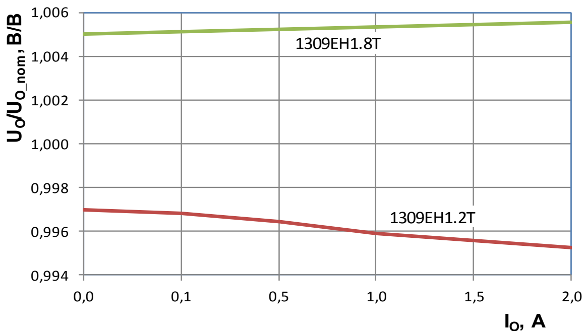
Рисунок 9 – Зависимость выходного напряжения U_o (приведенного к выходному напряжению номинальному U_{o\_nom} ) от тока нагрузки при U_i = 2,8 В для 1309EH1.2T и U_i = 2,6 В для 1309EH1.8T, T = 25 °C
