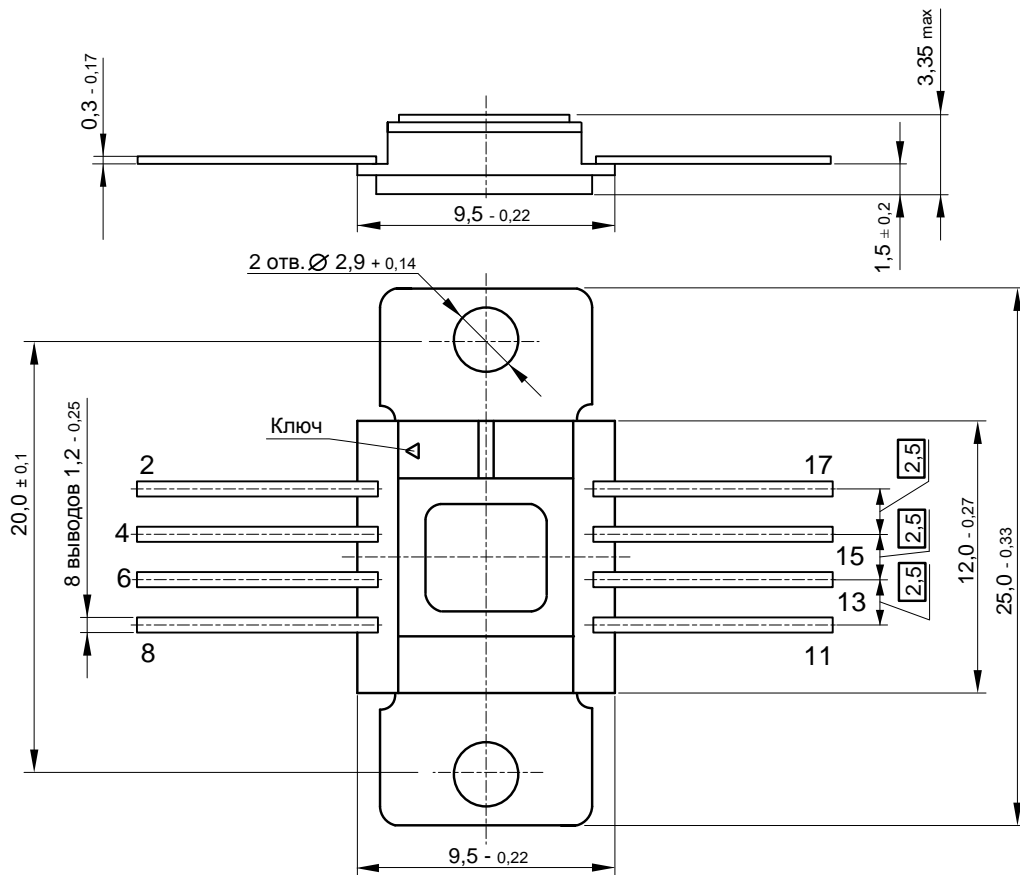
Рисунок 20 – Корпус 4116.8-3
