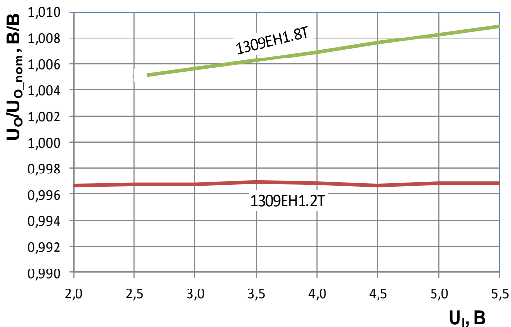
Рисунок 7 – Зависимость выходного напряжения U_o (приведенного к выходному напряжению номинальному U_{o\_nom} ) от входного напряжения при I_o = 100 мА, T = 25 °С
