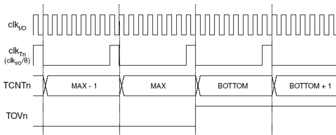
Рисунок 3.33 – Временная диаграмма таймера/счетчика с предделителем ( f_{clk\_I/O}/8 )
