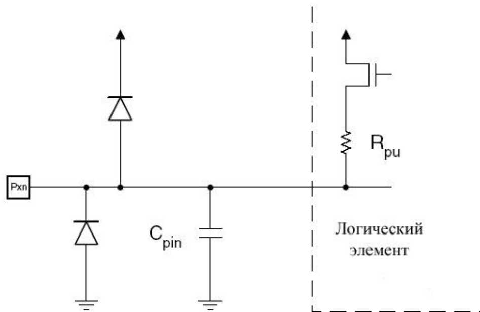
Рисунок 3.20 – Эквивалентная схема порта входа/выхода
