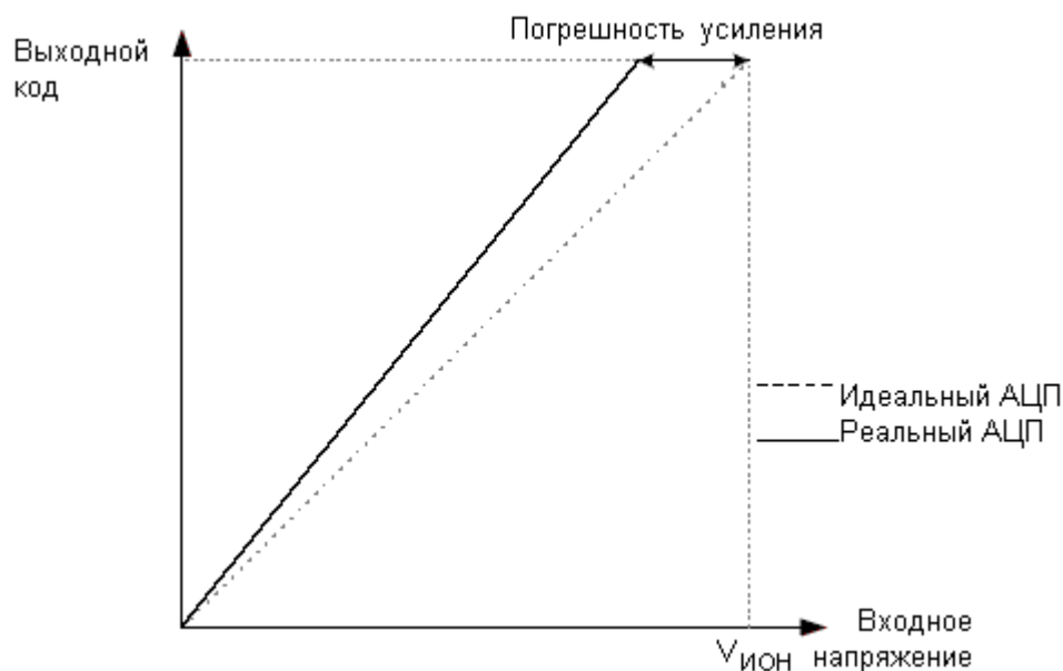
Рисунок 3.105 – Погрешность усиления
