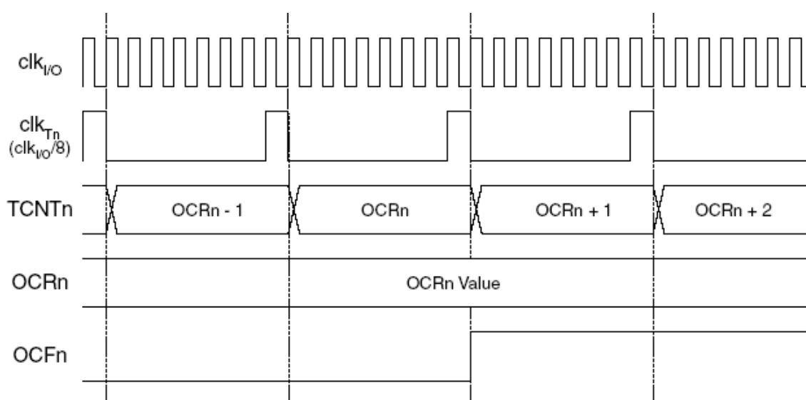
Рисунок 3.33 – Временная диаграмма таймера/счетчика с предделителем ( f_{clk\_I/O}/8 )
