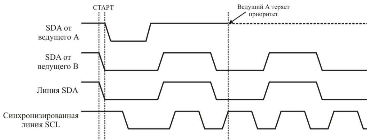
Рисунок 3.81 – Арбитраж двух ведущих
