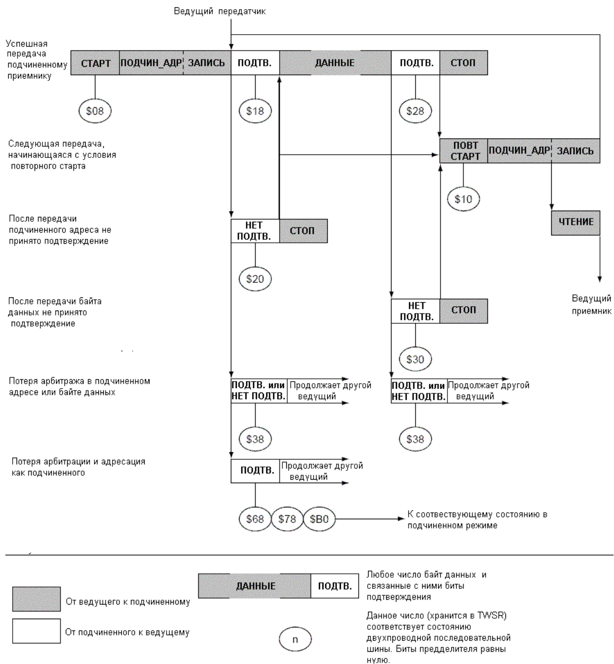
Рисунок 3.85 – Форматы и состояния в режиме ведущего передатчика
