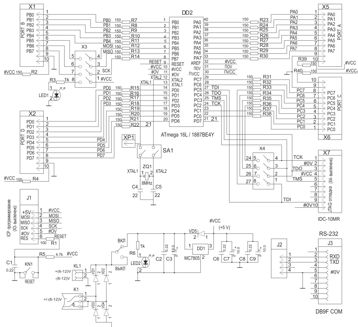
Рисунок В.1 – Схема электрическая основной платы с 40-выводной DIP-колодкой с нуле- вым усилением для установки микроконтроллеров 1887BE4Y / ATmega16 и макетным полем
