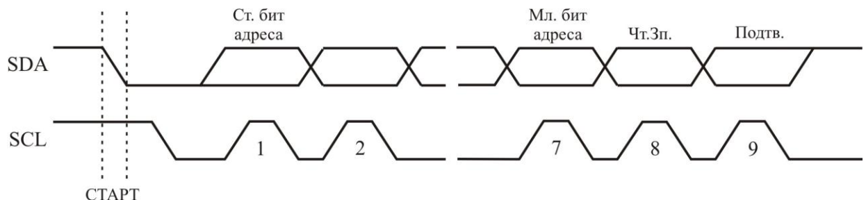
Рисунок 3.77 – Формат адресного пакета
