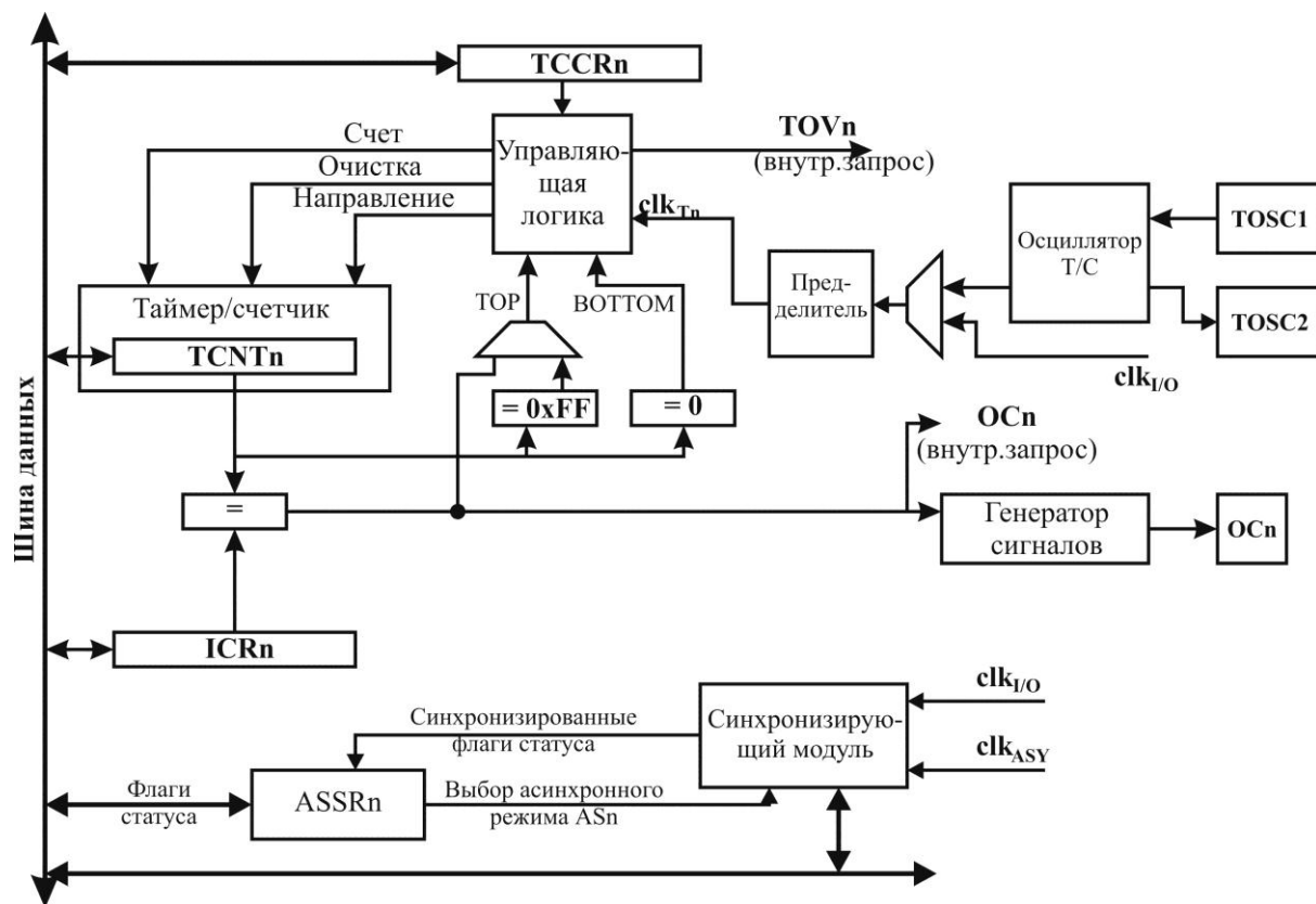
Рисунок 3.51 – Блок-схема 8-разрядного таймера/счетчика
