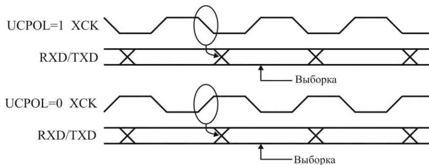
Рисунок 3.69 – Временная диаграмма для синхронного режима XCK
