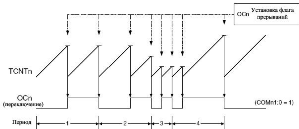
Рисунок 3.55 – Режим CTC, временная диаграмма
