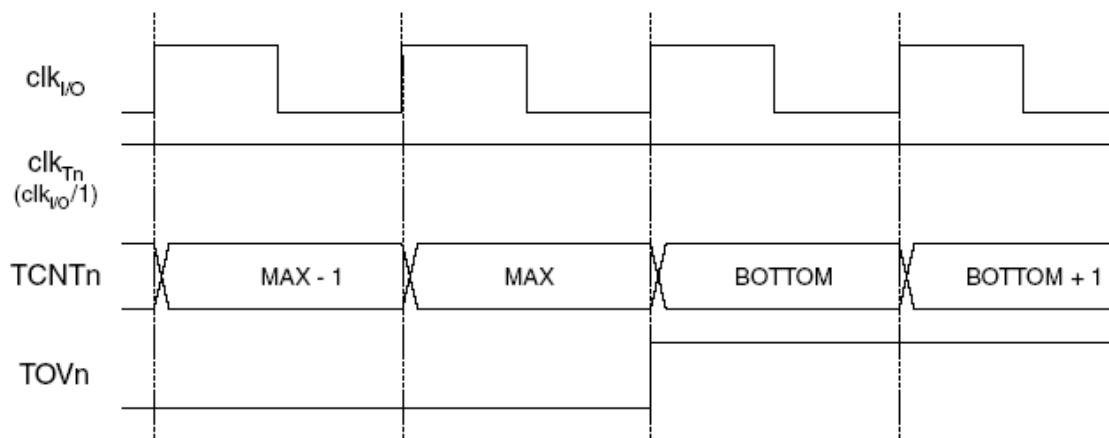
Рисунок 3.32 – Временная диаграмма таймера/счетчика без предделителя
