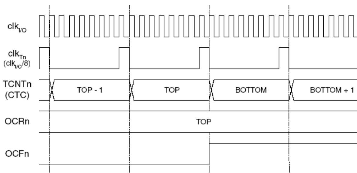
Рисунок 3.60 – Временная диаграмма таймера/счетчика с установкой OCF2 и предварительным делением частоты ( f_{clk\_I/O/8} )
