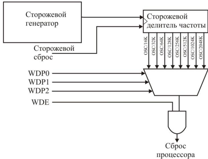
Рисунок 3.19 – Сторожевой таймер
