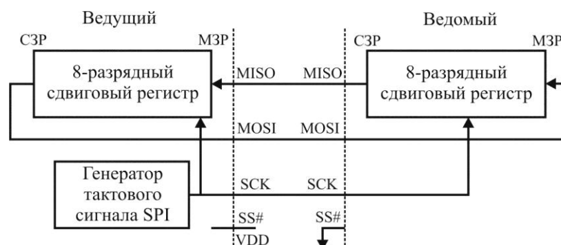
Рисунок 3.65 – Соединение микроконтроллеров по интерфейсу SPI
