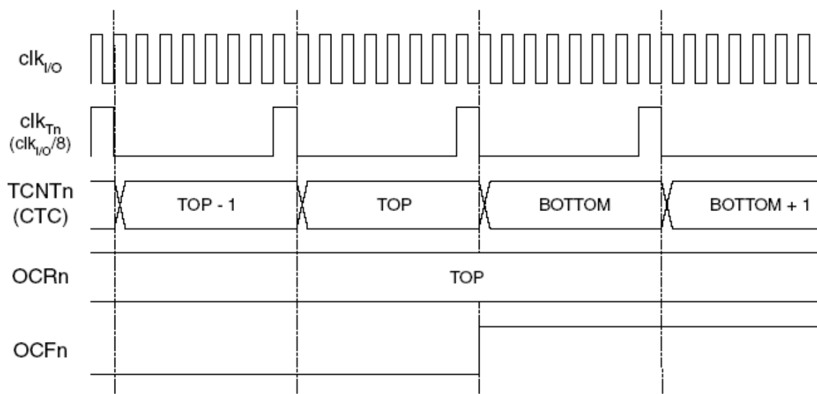
Рисунок 3.35 – Временная диаграмма таймера/счетчика, сброс таймера в режиме сравнения/совпадения, с предделителем ( f_{clk\_I/O}/8 )
