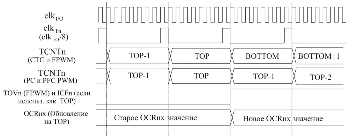
Рисунок 3.50 – Временная диаграмма таймера/счетчика с устройством предварительного деления частоты ( f_{clk\_I/O}/8 )
