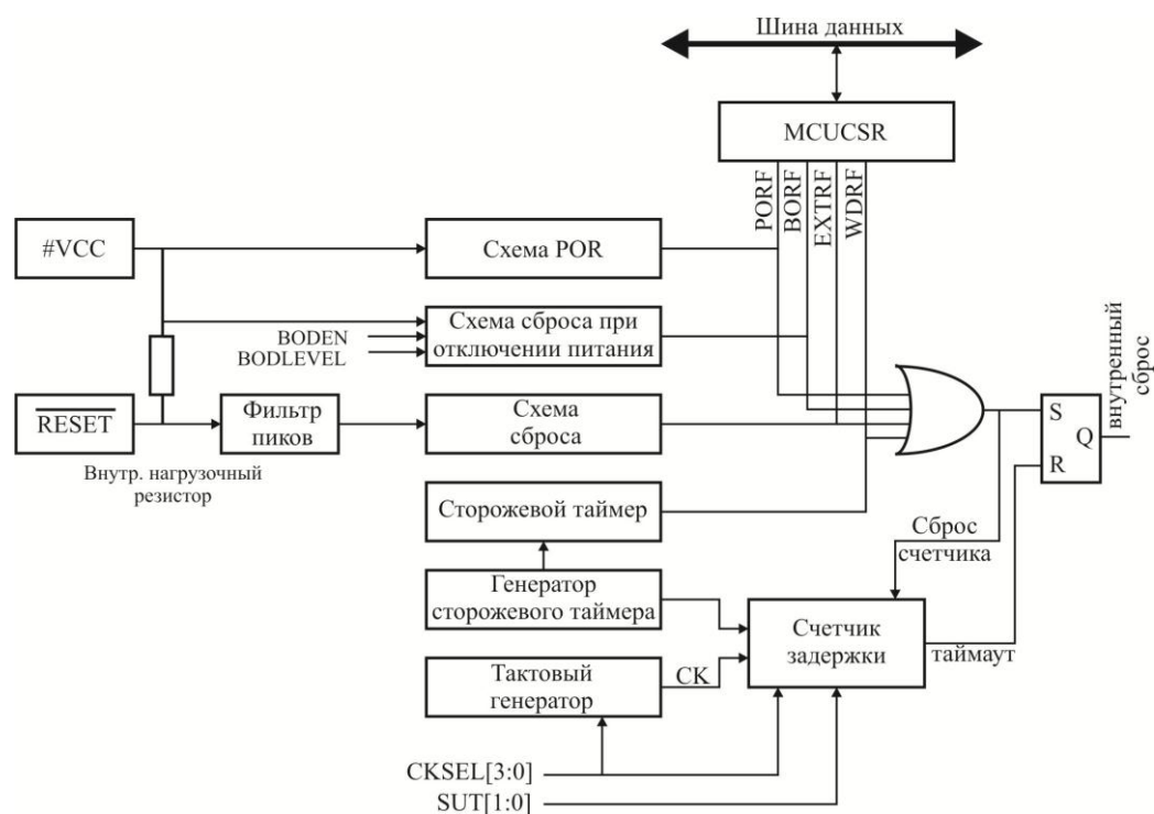
Рисунок 3.13 – Логика сброса
