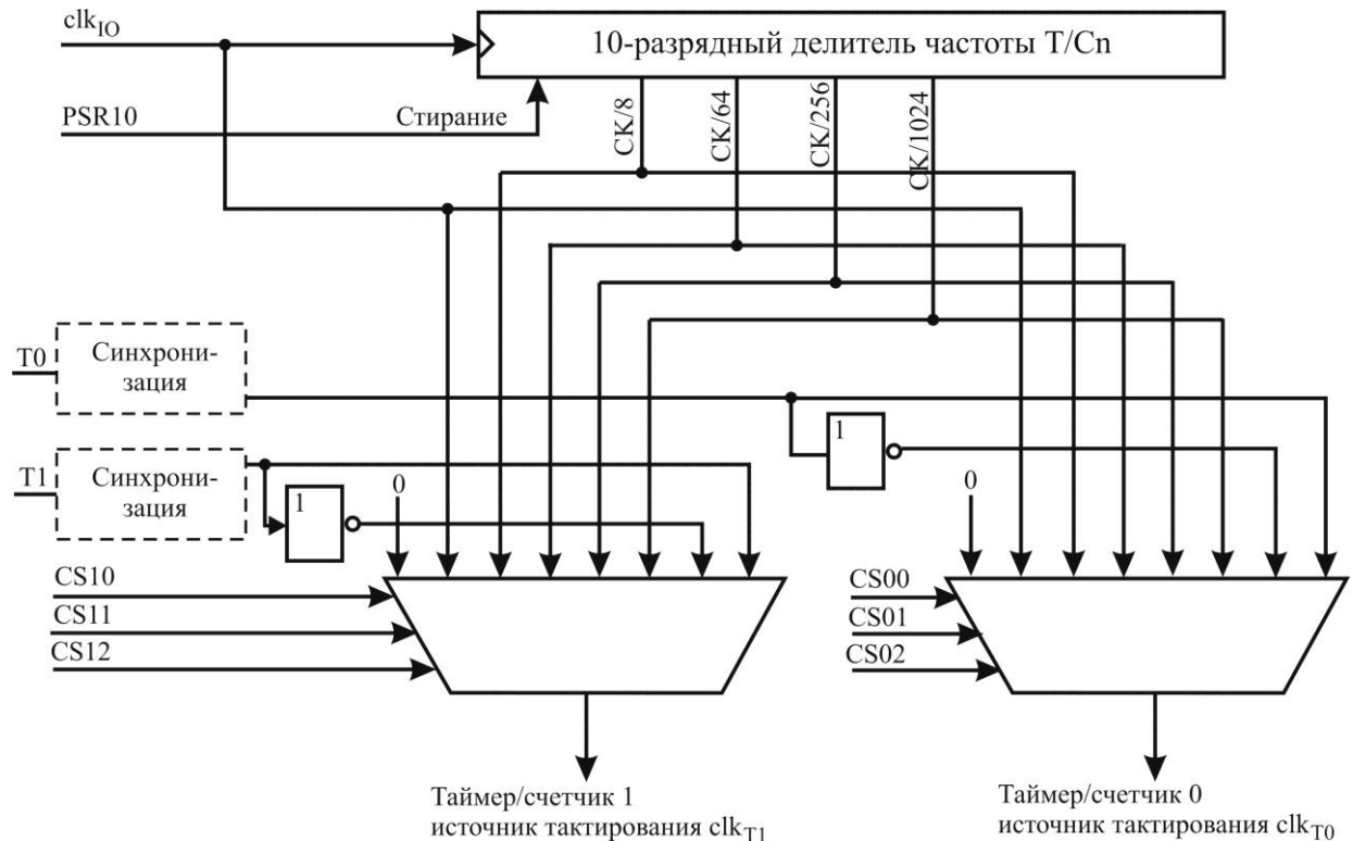
Рисунок 3.37 – Устройство предварительного деления частоты для таймера/счетчика 0 и таймера/счетчика 1
