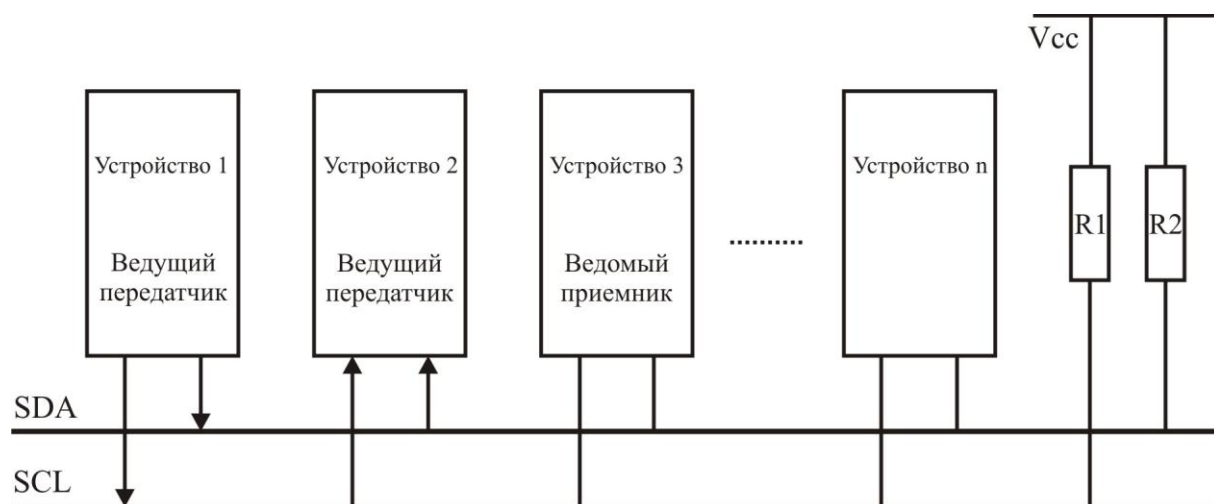
Рисунок 3.93 – Пример арбитража
