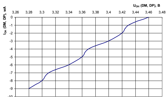
Рис. 65 Зависимость выходного напряжения высокого уровня на выводах DM, DP от тока нагрузки при: T=25^{\circ}\text{C} , U_{CC}=4,5 В
