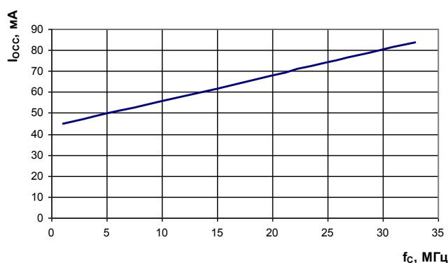
Рис. 63 Зависимость динамического тока потребления от частоты следования синхроимпульсов ( f_c ), при: T=25^{\circ}\text{C} , U_{CC}=5,5 В, f_{USB}=48 МГц
