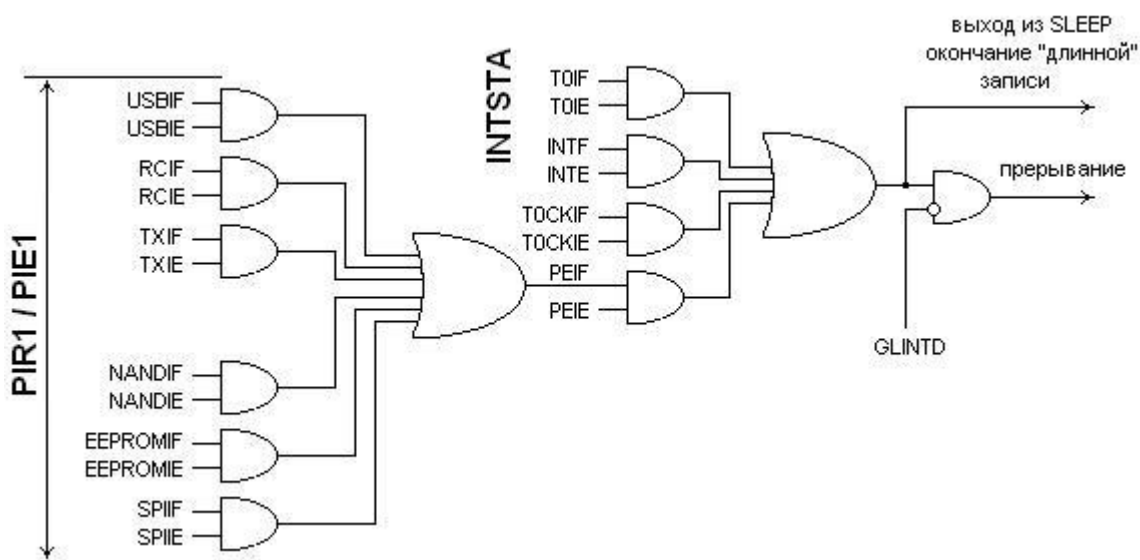
Рис. 10 Структурная схема логики прерываний
