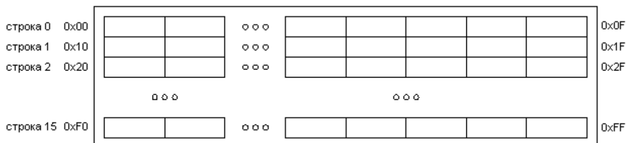
Рис. 40 Структурная схема организации EEPROM памяти
