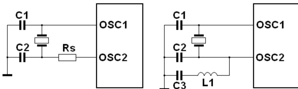
Рис. 1 Подключение резонатора.
