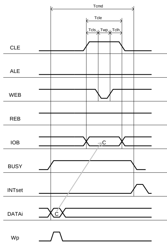
Рис. 48 Диаграмма сигналов записи команды в NAND Flash память
