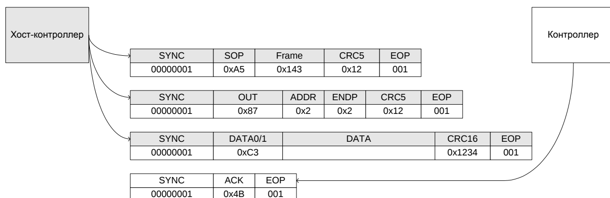
Рис. 58 Режим передачи OUT
