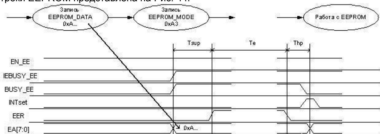
Рис. 44 Стирание строки EEPROM памяти
