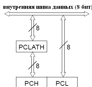
Рис. 16 Функционирование счётчика команд
