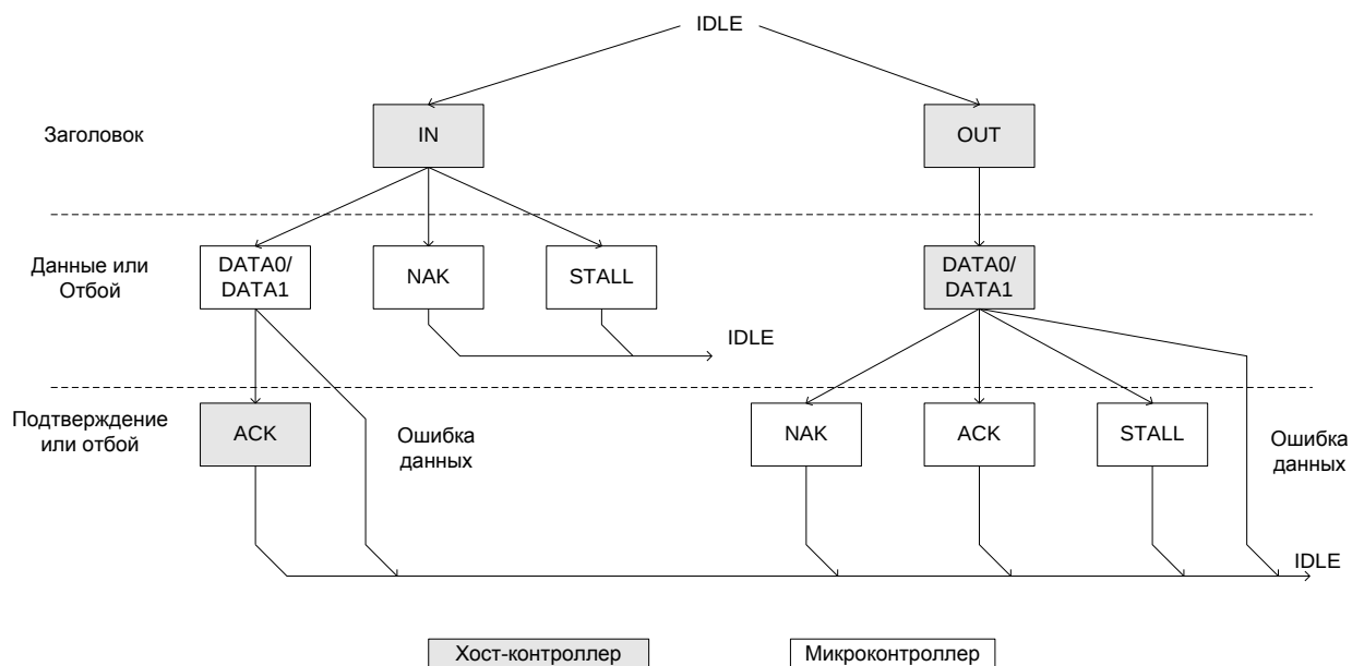
Рис. 60 Тип обмена Bulk Transaction
