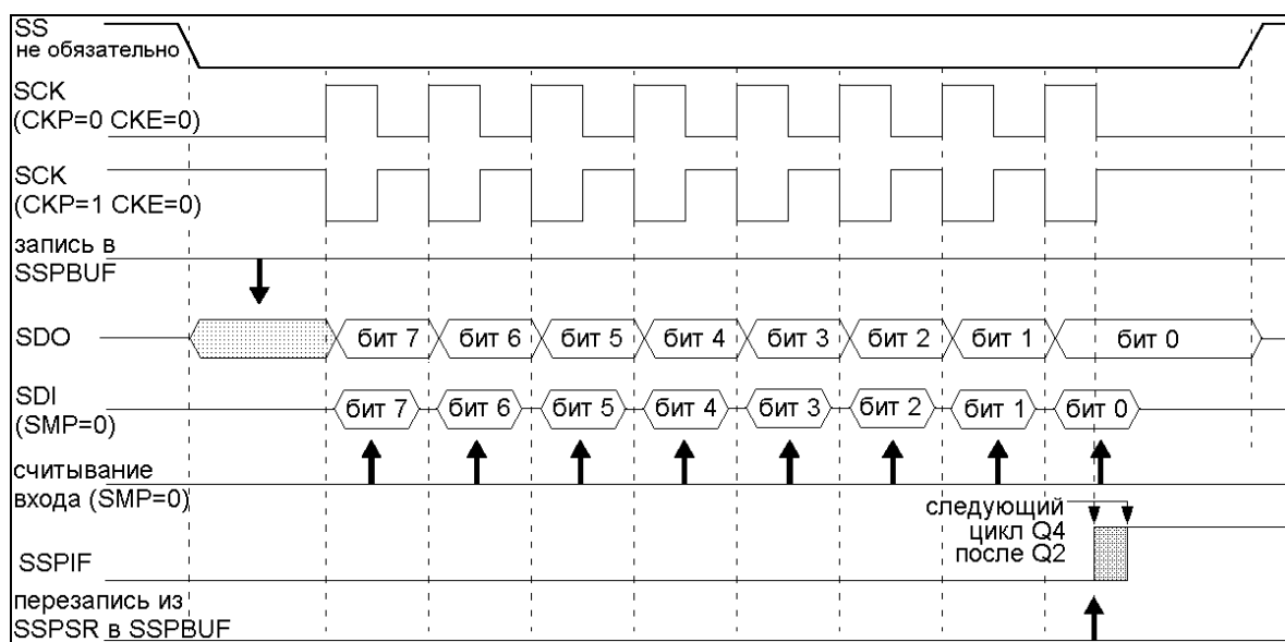
Рис. 30 Работа модуля SPI в режиме ведомый (CKE = 0)
