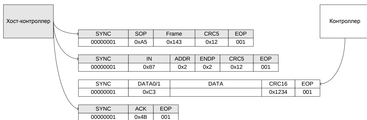
Рис. 57 Режим передачи IN
