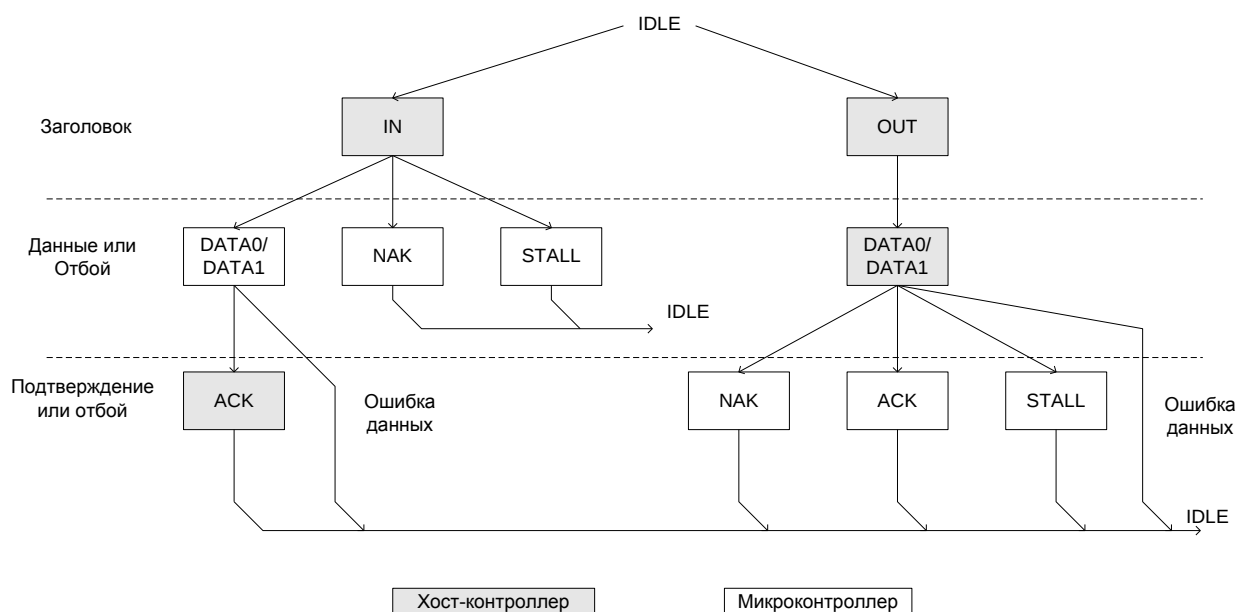
Рис. 59 Тип обмена Interrupt Transaction
