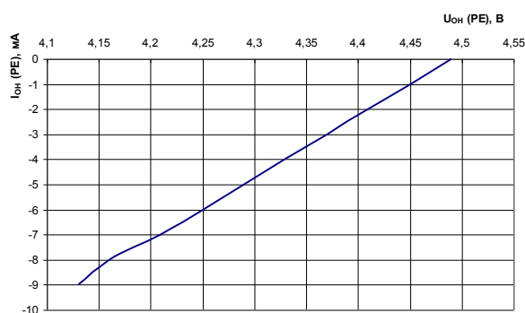
Рис. 77 Зависимость выходного напряжения высокого уровня на выводах РЕ от тока нагрузки при: T = 25^{\circ}\text{C} , U_{CC} = 4,5 \text{ В}
