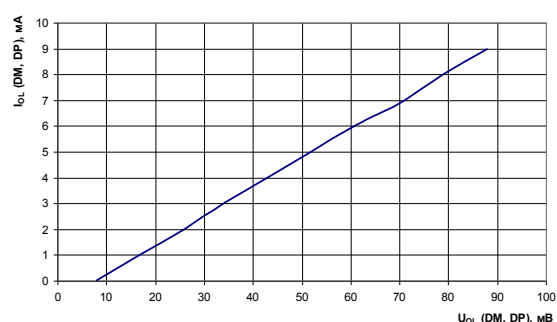
Рис. 66 Зависимость выходного напряжения низкого уровня на выводах DM, DP от тока нагрузки при: T=25^{\circ}\text{C} , U_{CC}=4,5 В
