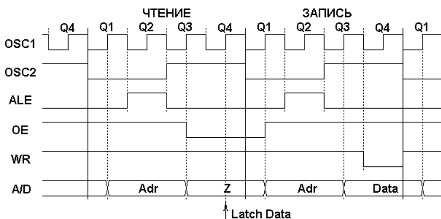
Рис. 14 Диаграммы сигналов доступа к внешней памяти программ
