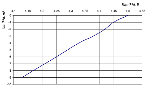
Рис. 67 Зависимость выходного напряжения высокого уровня на выводах PA от тока нагрузки при: T = 25^{\circ}\text{C} , U_{CC} = 4,5 \text{ В}
