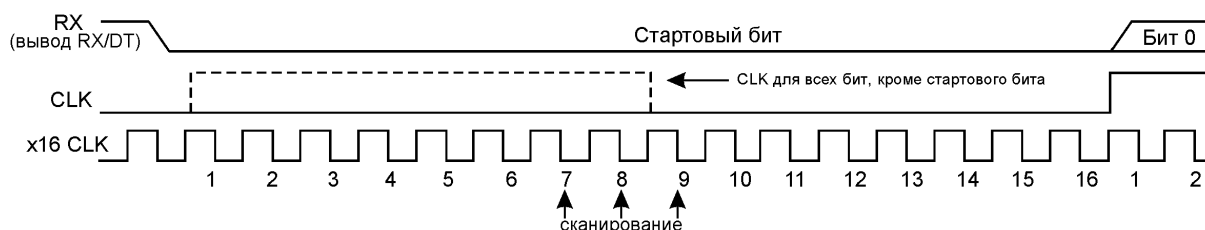
Рис. 36 Схема сканирования вывода PA2/RX/DT
