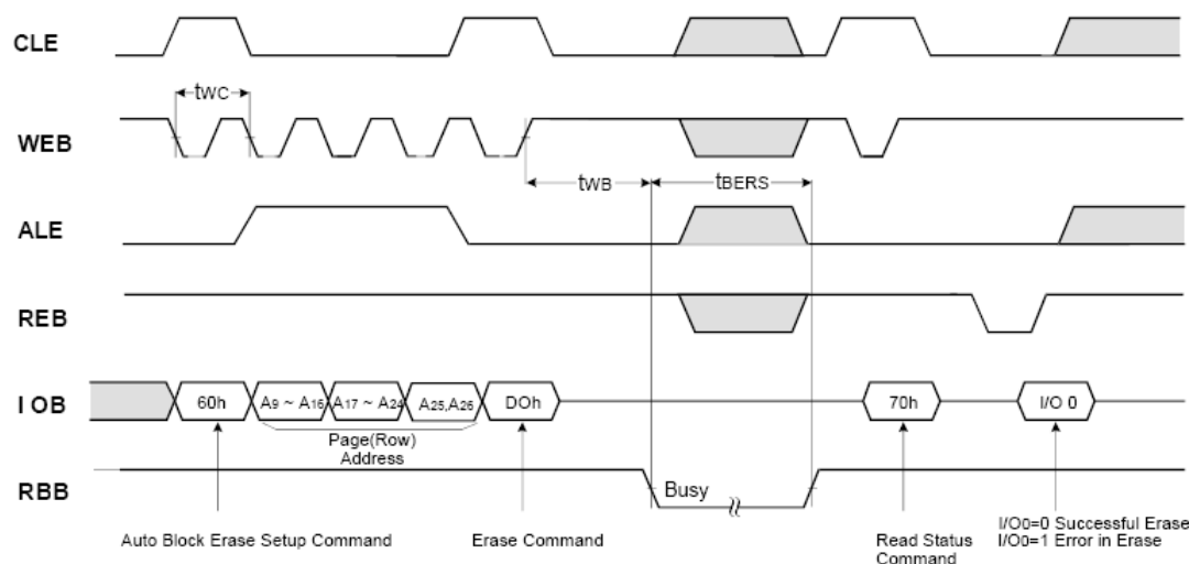
Рис. 50 Диаграмма сигналов при стирании страницы NAND Flash памяти
