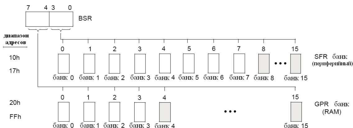
Рис. 18 Функционирование BSR
