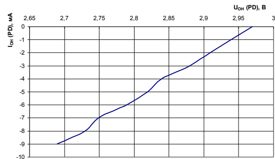
Рис. 70 Зависимость выходного напряжения высокого уровня на выводах PD от тока нагрузки при: T = 25^{\circ}\text{C} , U_{CC} = 4,5 \text{ В} , U_{CCP} = 3,0 \text{ В}
