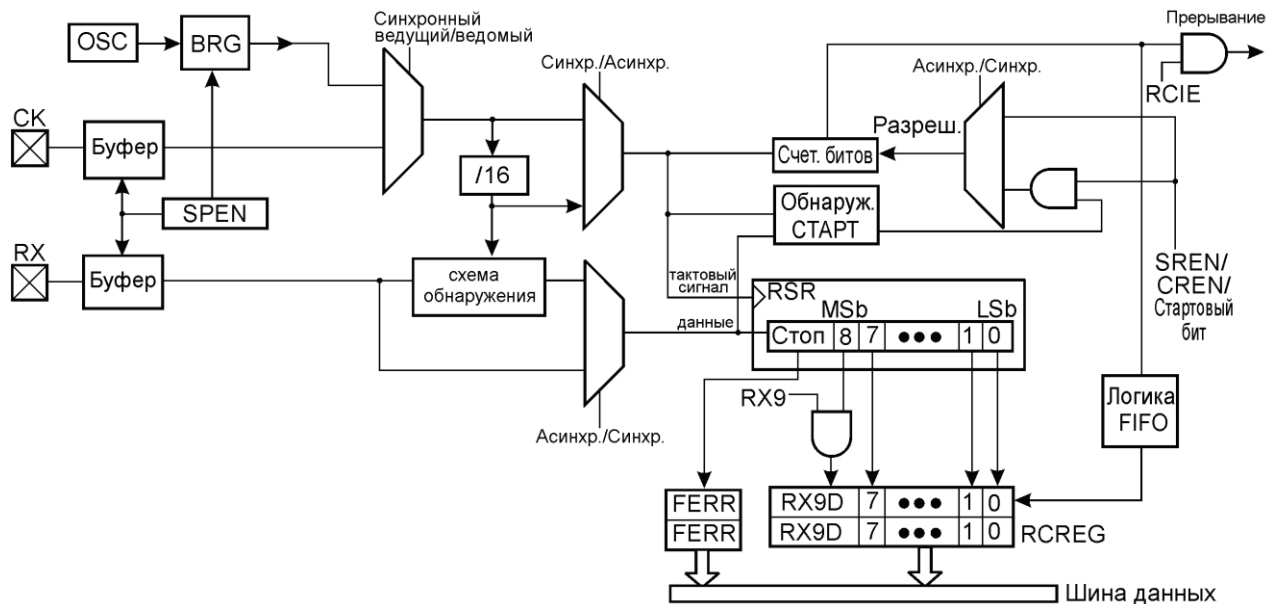
Рис. 33 Блок-схема приемника
