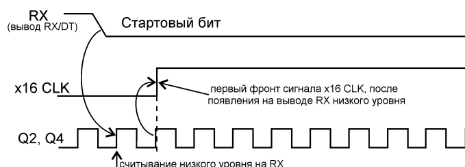
Рис. 37 Обнаружение стартового бита
