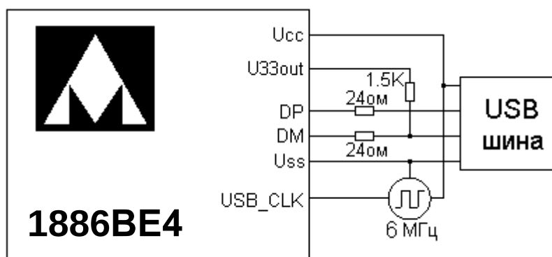
Рис. 54 Схема подключения микроконтроллера к USB шине в режиме Low Speed
