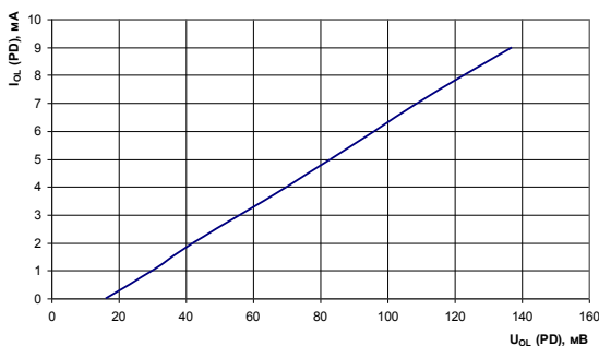
Рис. 71 Зависимость выходного напряжения низкого уровня на выводах PD от тока нагрузки при: T = 25^{\circ}\text{C} , U_{CC} = 4,5 \text{ В} , U_{CCP} = 3,0 \text{ В}
