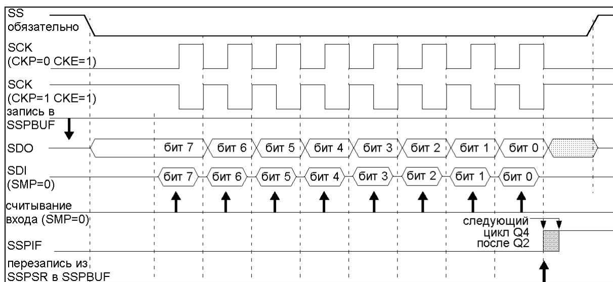
Рис. 31 Работа модуля SPI в режиме ведомый (CKE = 1)
