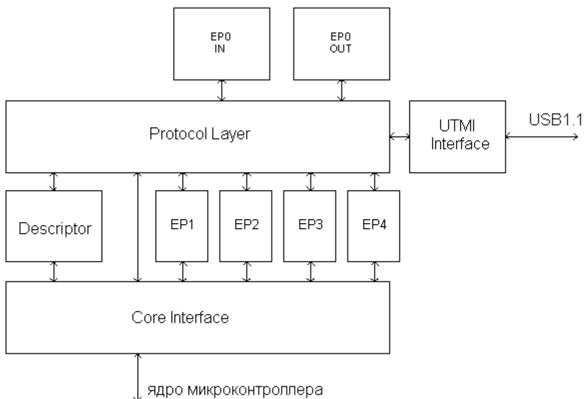
Рис. 55 Структурная схема блока USB
