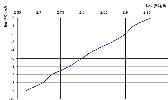
Рис. 74 Зависимость выходного напряжения высокого уровня на выводах РС от тока нагрузки при: T = 25^{\circ}\text{C} , U_{CC} = 4,5 \text{ В} , U_{CCP} = 3,0 \text{ В}
