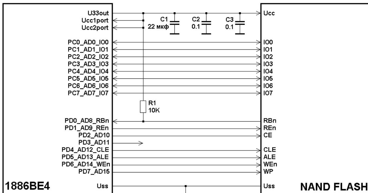
Рис. 47 Подключение к микроконтроллеру внешней NAND Flash памяти
