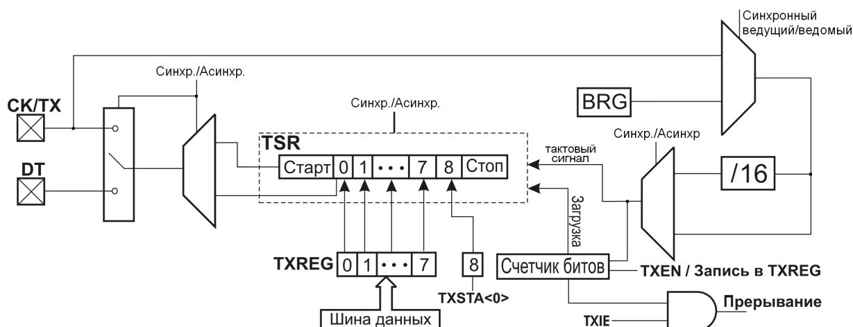
Рис. 32 Блок-схема передатчика
