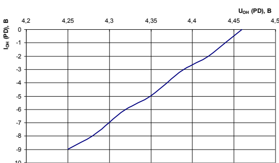
Рис. 69 Зависимость выходного напряжения высокого уровня на выводах PD от тока нагрузки при: T = 25^{\circ}\text{C} , U_{CC} = 4,5 \text{ В} , U_{CCP} = 4,5 \text{ В}
