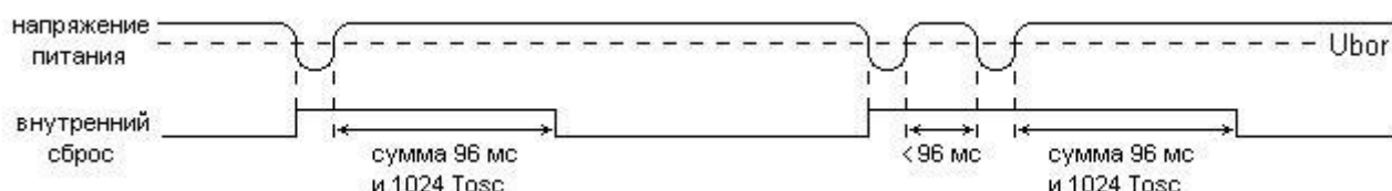
Рис. 9 Сброс по снижению напряжения питания
