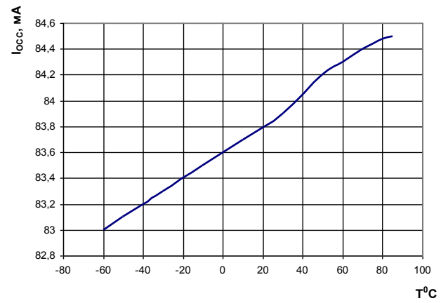
Рис. 80 Зависимость динамического тока потребления от температуры U_{\text{CC}} = 5,5 \text{ В} , f_{\text{с}} = 33 \text{ МГц} , f_{\text{USB}} = 48 \text{ МГц}
