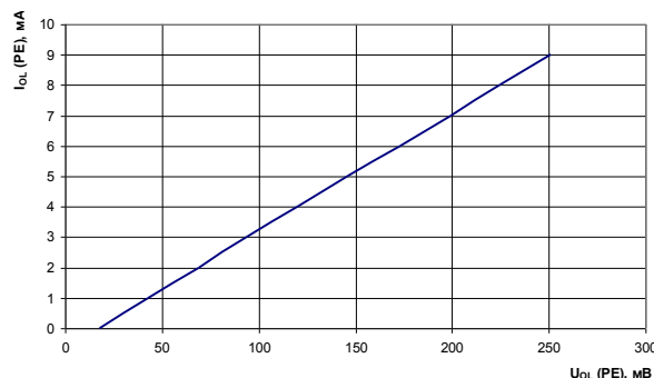
Рис. 78 Зависимость выходного напряжения низкого уровня на выводах РЕ от тока нагрузки при: T = 25^{\circ}\text{C} , U_{CC} = 4,5 \text{ В}
