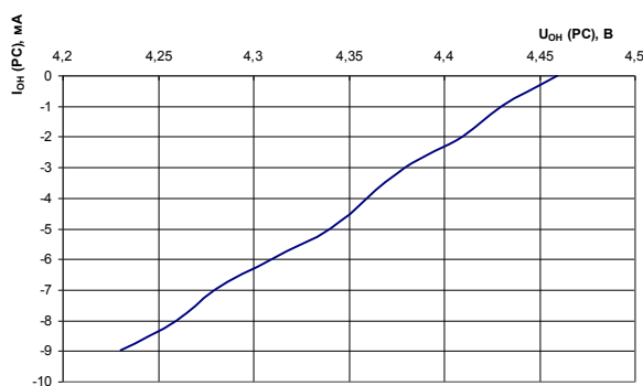
Рис. 73 Зависимость выходного напряжения высокого уровня на выводах РС от тока нагрузки при: T = 25^{\circ}\text{C} , U_{CC} = 4,5 \text{ В} , U_{CCP} = 4,5 \text{ В}
