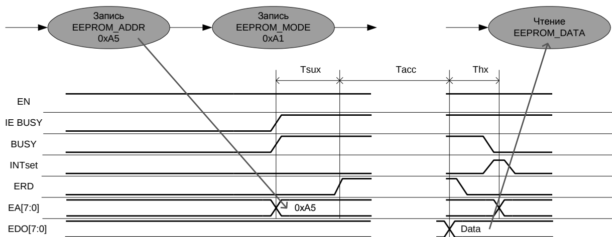
Рис. 46 Чтение байта из EEPROM памяти
