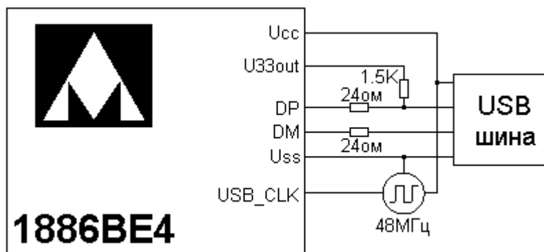
Рис. 53 Схема подключения микроконтроллера к USB шине в режиме Full Speed
