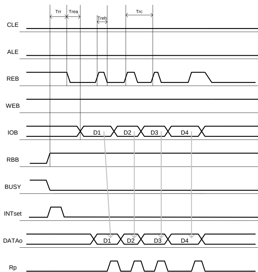
Рис. 52 Диаграмма сигналов чтения данных из NAND Flash памяти
