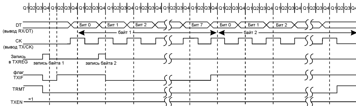
Рис. 38 Синхронная передача в ведущем режиме
