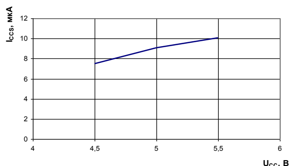
Рис. 64 Зависимость статического тока потребления от напряжения питания при: T=25^{\circ}\text{C}
