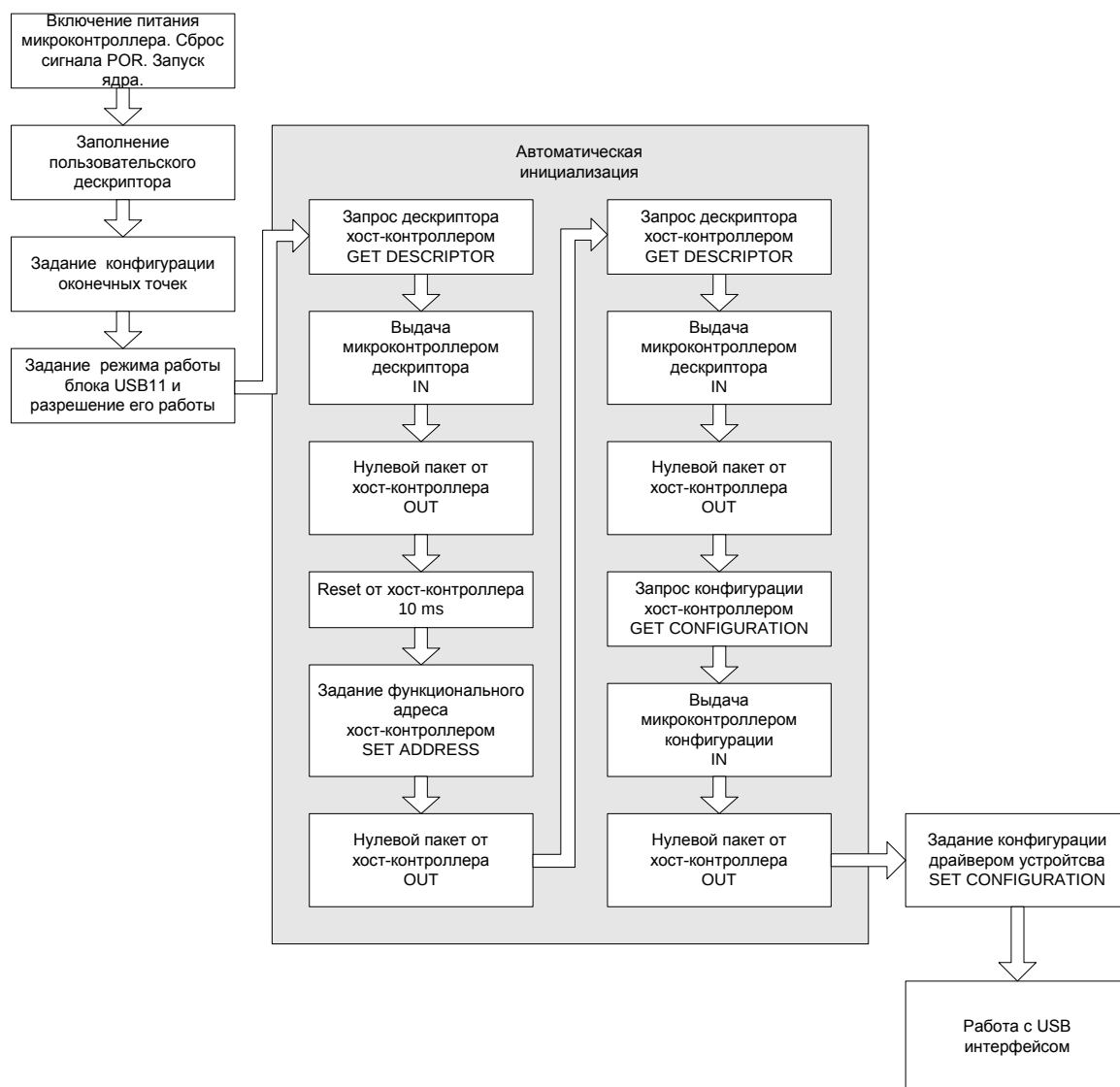
Рис. 56 Блок-схема работы микроконтроллера при запуске USB интерфейса
