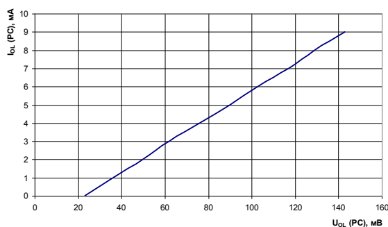
Рис. 75 Зависимость выходного напряжения низкого уровня на выводах РС от тока нагрузки при: T = 25^{\circ}\text{C} , U_{CC} = 4,5 \text{ В} , U_{CCP} = 3,0 \text{ В}
