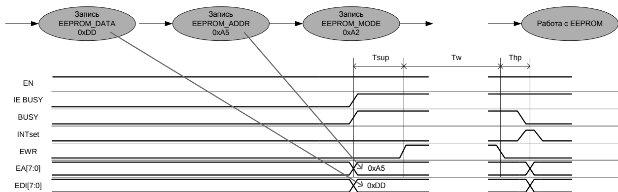
Рис. 45 Запись байта в EEPROM память
