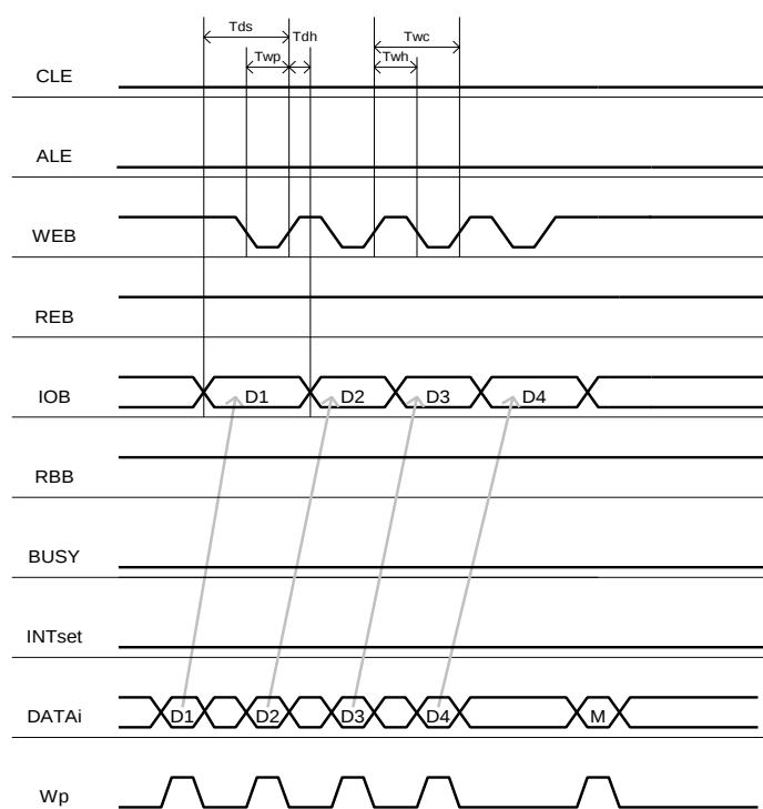
Рис. 51 Диаграмма сигналов записи данных в NAND Flash память
