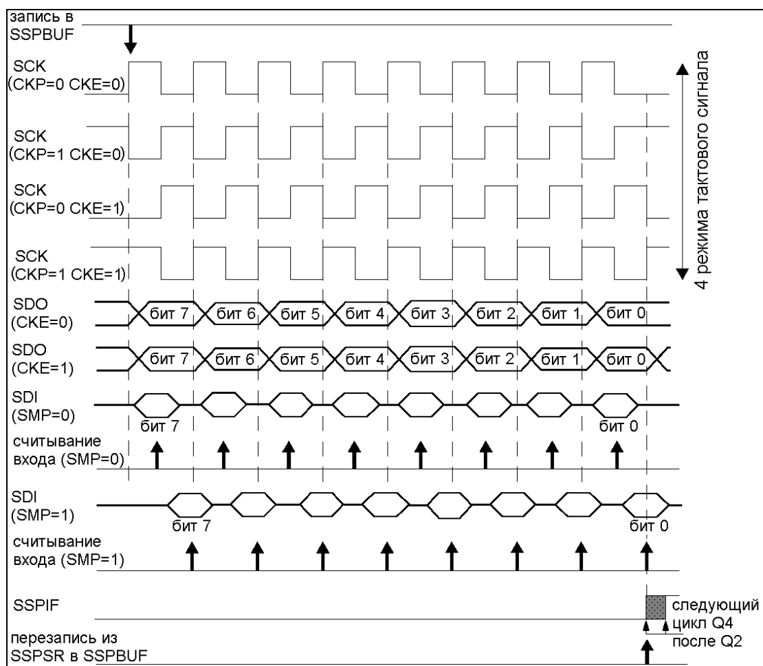
Рис. 28 Работа модуля SPI в режиме ведущего
