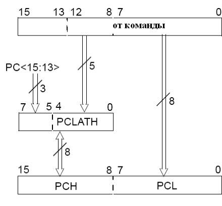
Рис. 17 Счетчик команд при выполнении инструкций CALL и GOTO
