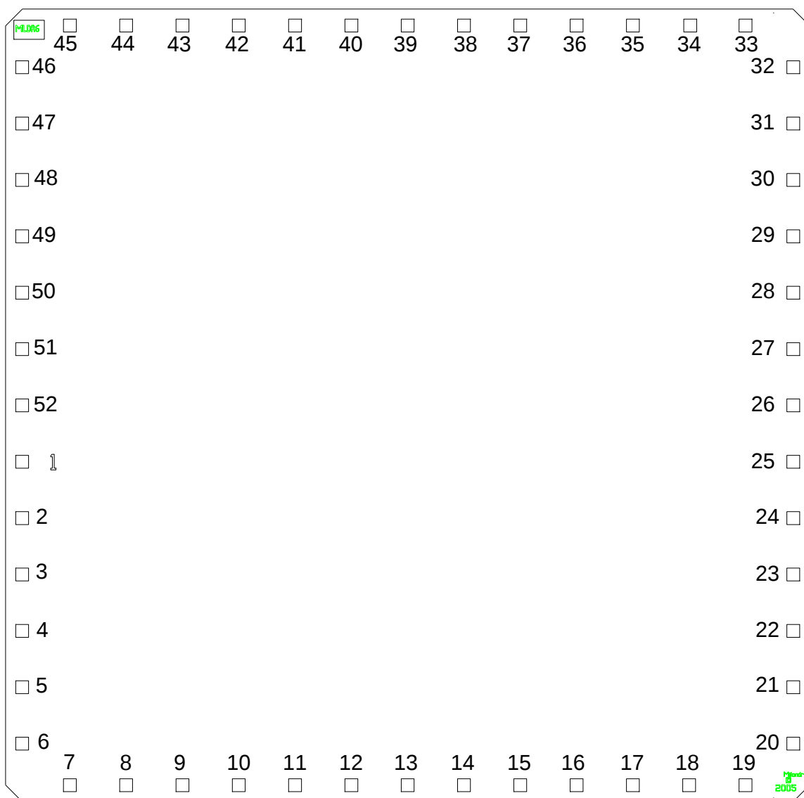
Рис. 82 Кристалл 6,25 max x 6,35 max (мм)
