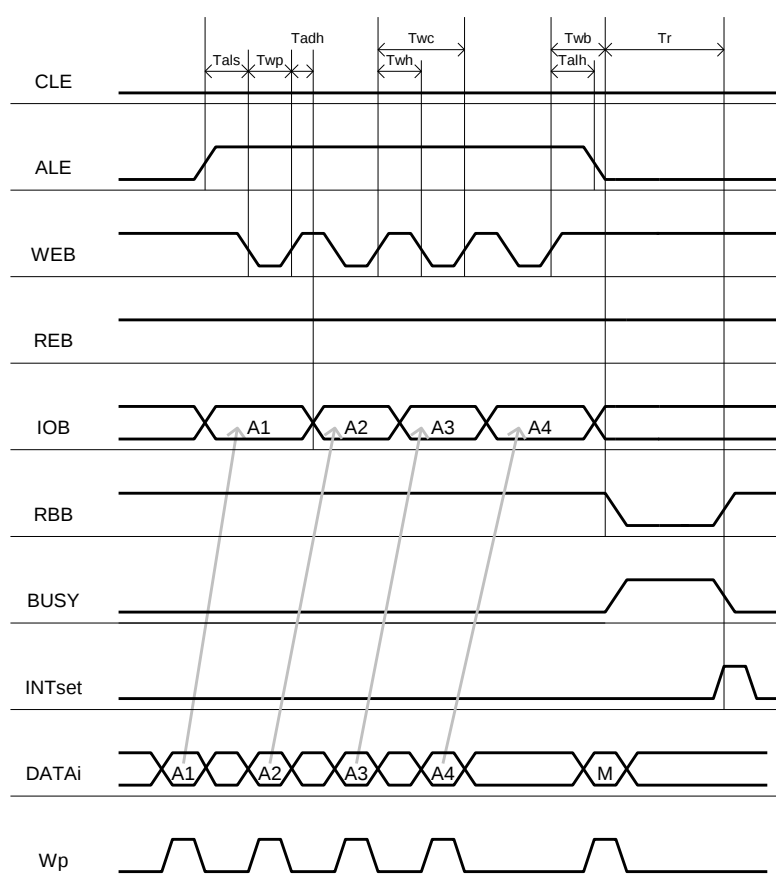
Рис. 49 Диаграмма сигналов записи адреса в NAND Flash память
