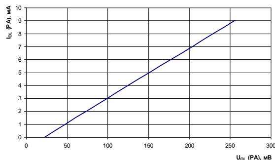
Рис. 68 Зависимость выходного напряжения низкого уровня на выводах PA от тока нагрузки при: T = 25^{\circ}\text{C} , U_{CC} = 4,5 \text{ В}
