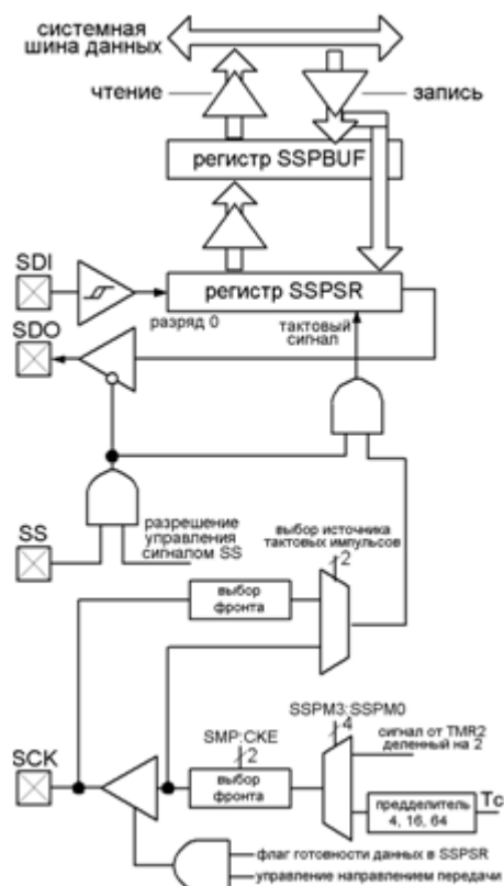
Рис. 27 Блок-схема модуля SPI
