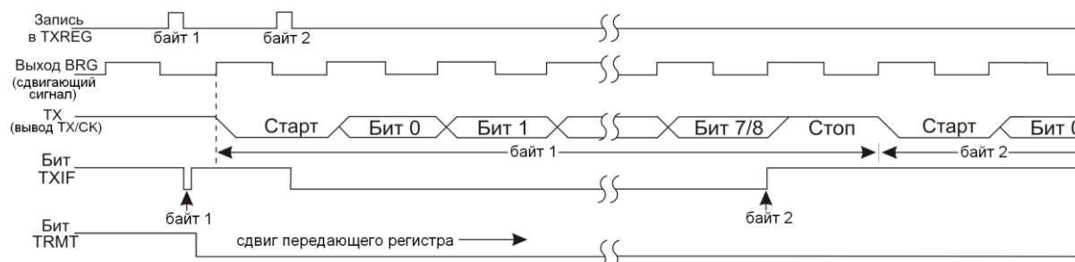
Рис. 35 Асинхронная неразрывная последовательная передача
