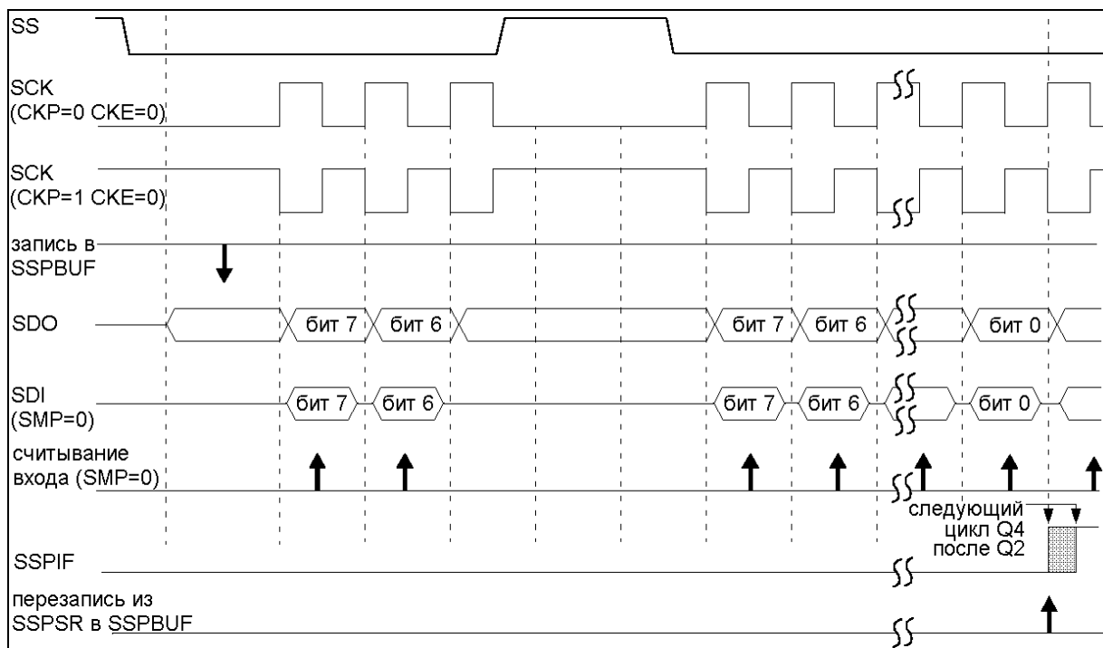
Рис. 29 Демонстрация работы в режиме синхронного ведомого
