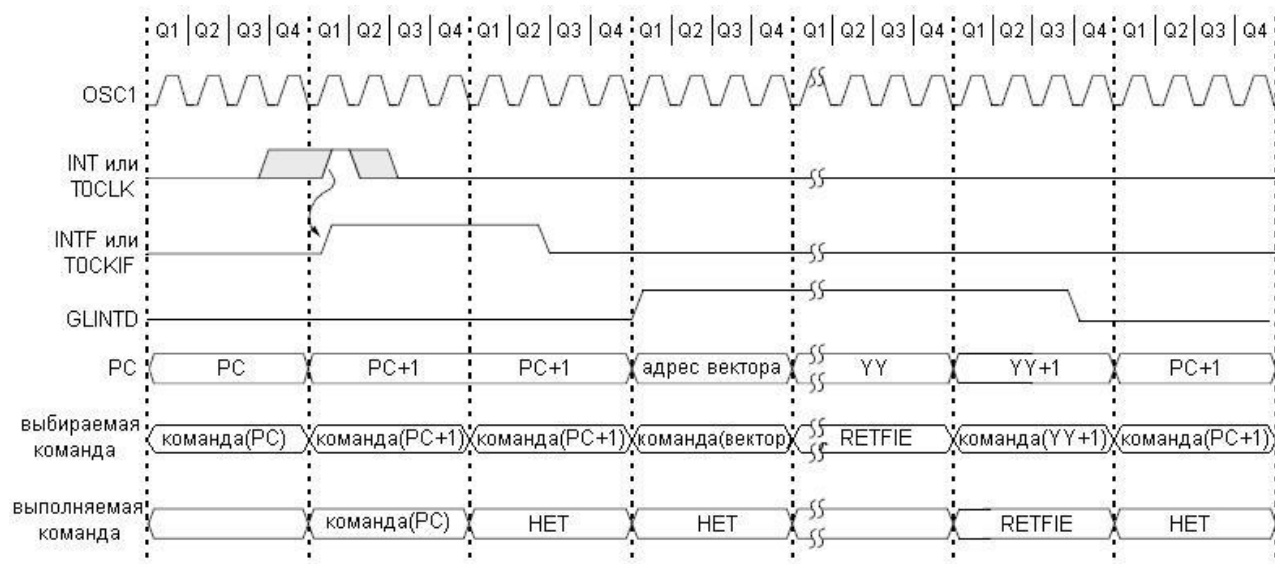
Рис. 11 Временная диаграмма обработки прерываний от выводов PA0/INT или PA1/T0CLK
