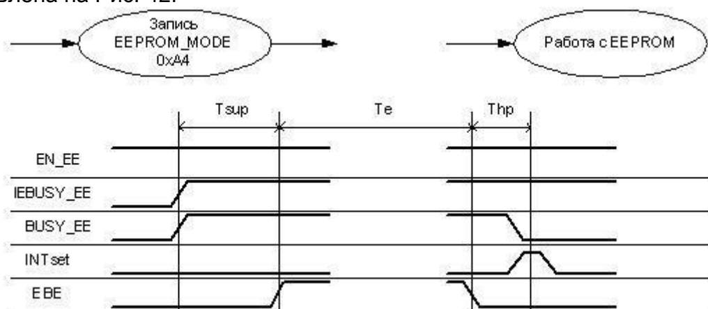
Рис. 42 Стирание всей EEPROM памяти в TEST режиме
