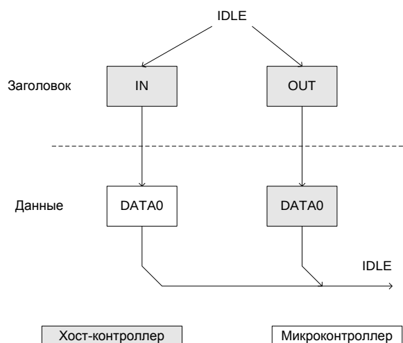
Рис. 61 Тип обмена Isochronous Transaction
