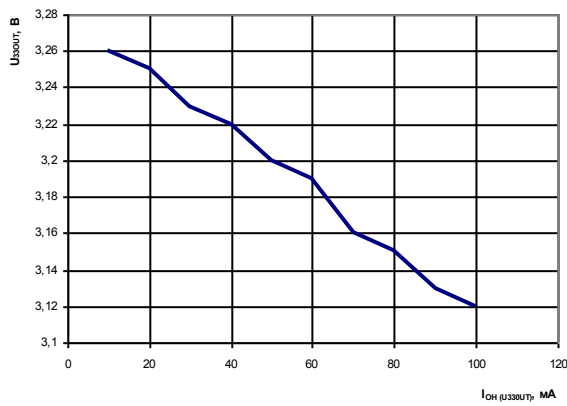
Рис. 79 Зависимость уровня внутреннего регулятора напряжения от тока нагрузки при: T = 25^\circ\text{C} , U_{\text{CC}} = 4,5 \text{ В}
