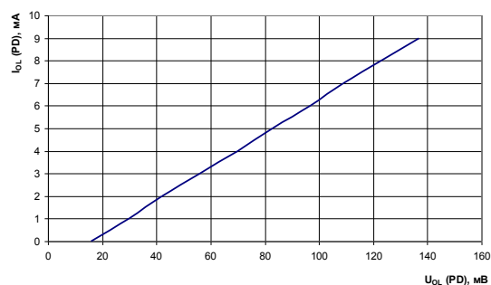
Рис. 72 Зависимость выходного напряжения низкого уровня на выводах PD от тока нагрузки при: T = 25^{\circ}\text{C} , U_{CC} = 4,5 \text{ В} , U_{CCP} = 4,5 \text{ В}
