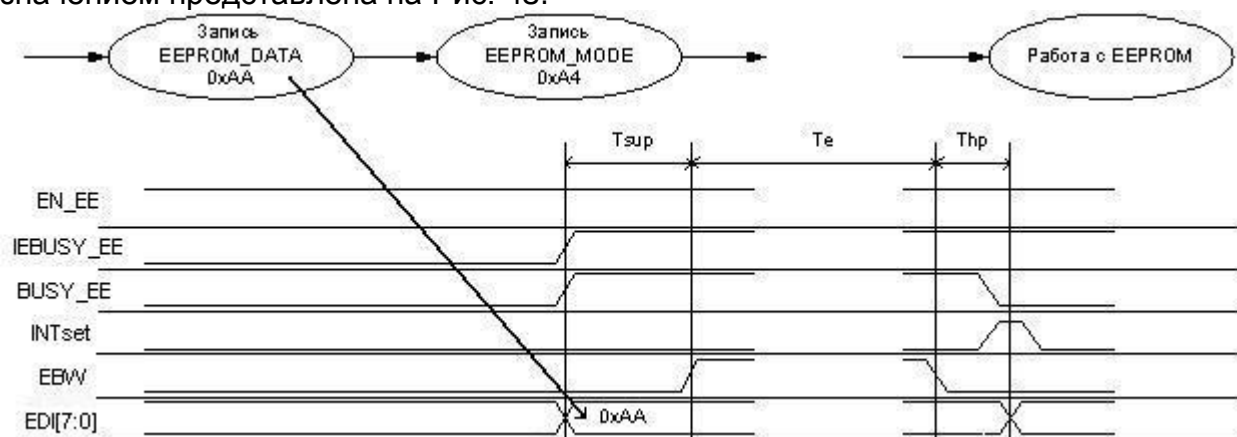
Рис. 43 Запись всей EEPROM памяти одним значением
