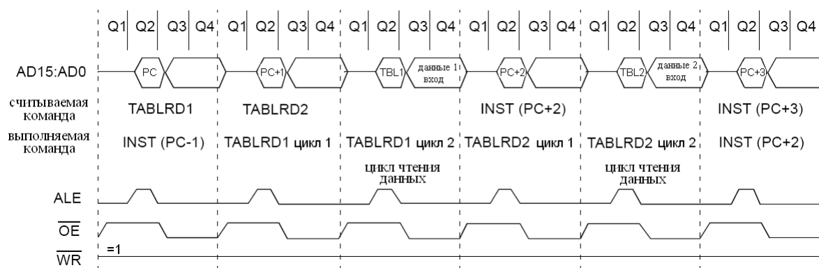
Рис. 23 Временная диаграмма последовательности команд TABLRD (внешняя память программ)
