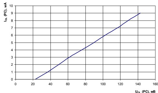
Рис. 76 Зависимость выходного напряжения низкого уровня на выводах РС от тока нагрузки при: T = 25^{\circ}\text{C} , U_{CC} = 4,5 \text{ В} , U_{CCP} = 4,5 \text{ В}
