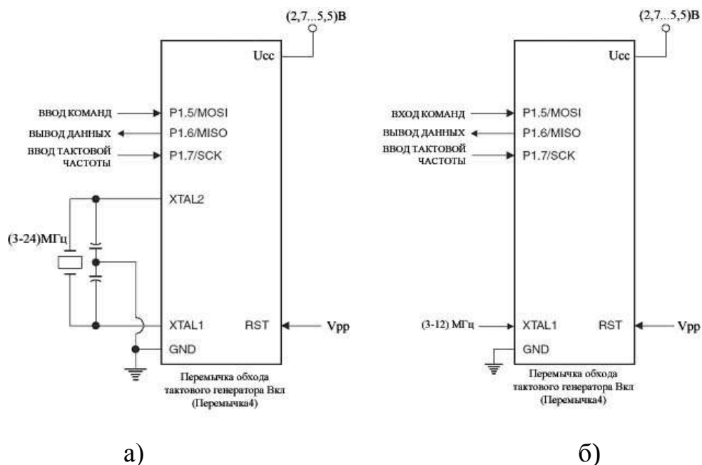
Рисунок 13 - Схема включения микросхемы при последовательном программировании: а) – с кварцевым резонатором;
