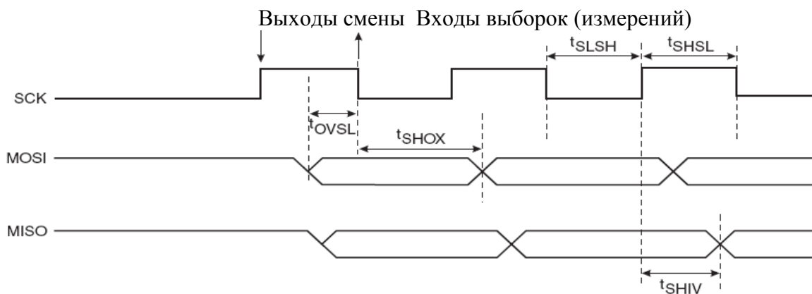
Рисунок 14 - Временные диаграммы при последовательном программировании
