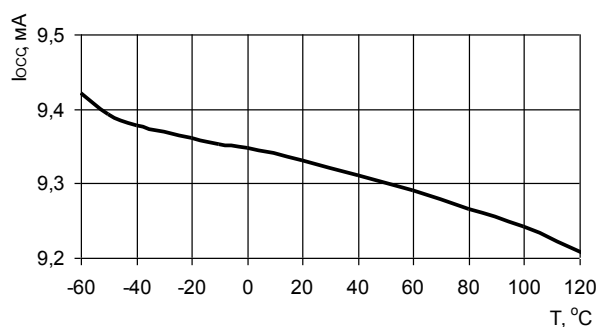
Рисунок 13 Зависимость динамического тока потребления от температуры, при: U_{CC} = 3,3\text{ В} , f_{EXCLK} = 33\text{ МГц}
