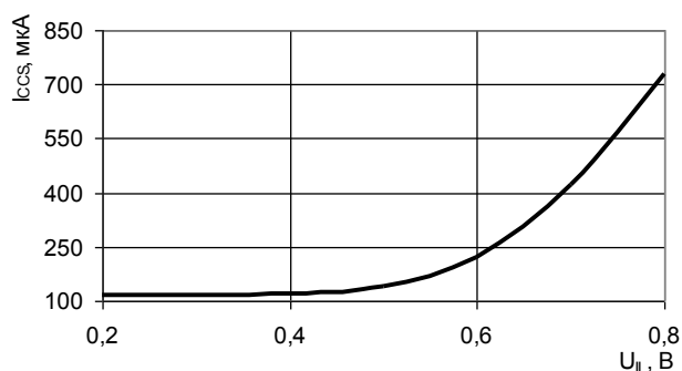
Рисунок 10 Зависимость тока потребления в режиме хранения от входного напряжения низкого уровня, при: U_{CC}=3,3\text{ В} , U_{IH}=2,2\text{ В} , T=25\text{ }^{\circ}\text{C}
