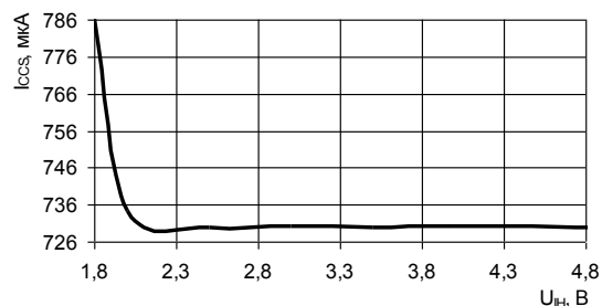
Рисунок 9 Зависимость тока потребления в режиме хранения от входного напряжения высокого уровня, при: U_{CC} = 3,3\text{ В} , U_{IL} = 0,8\text{ В} , T=25\text{ }^{\circ}\text{C}
