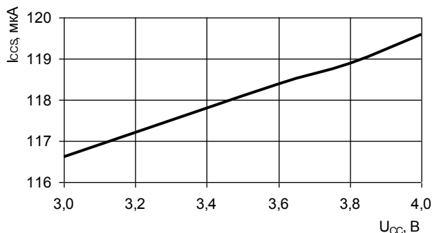
Рисунок 8 Зависимость тока потребления в режиме хранения, от напряжения питания, при: T=25\text{ }^{\circ}\text{C}
