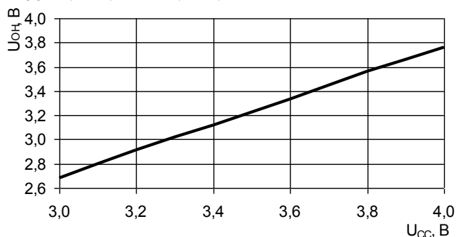
Рисунок 12 Зависимость выходного напряжения высокого уровня от напряжения питания, при: I_{OH}=\text{минус } 4\text{ мА} , T=25\text{ }^{\circ}\text{C}
