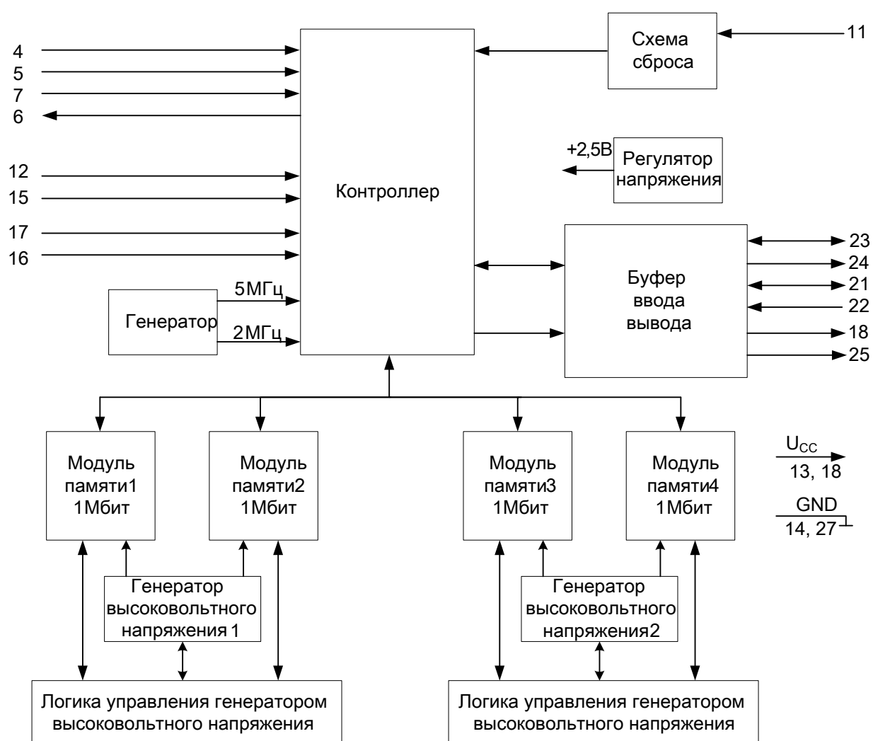
Рисунок 1 Структурная блок-схема
