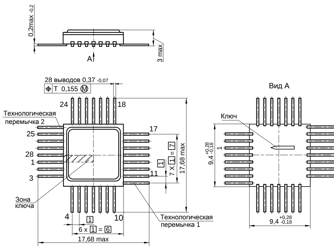
Рисунок 18 Корпус Н09.28-1В
