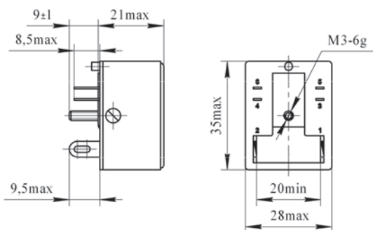
РЕЛЕ НА НОМИНАЛЬНЫЕ ТОКИ 0,5 ... 25,0 А С ДВУМЯ ЗАМЫКАЮЩИМИ ЦЕПЯМИ
